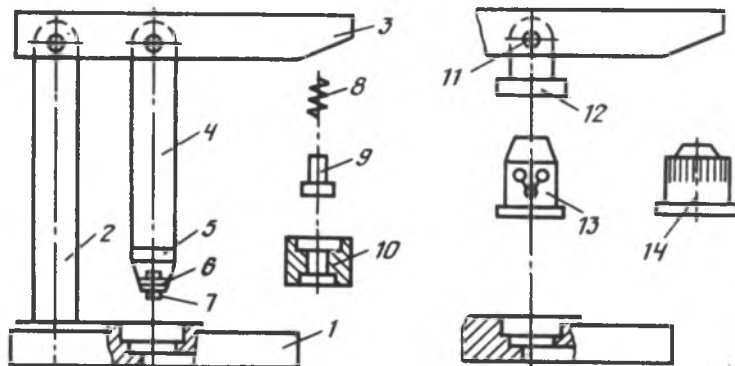
Прибор для снаряжения охотничьих патронов.
