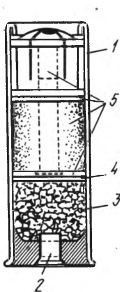
Пуля Ширинского-Шихматова. Первый образец.
