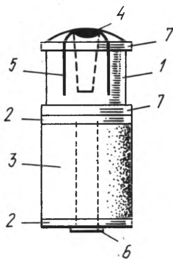
Усовершенствованная пуля (второй образец) Ширинского-Шихматова: 1 — свинцовый корпус пули; 2 — картонные прокладки; 3 — войлочный пыж; 4 — экспрессная пустота; 5 — надрезы, облегчающие разворачивание пули при ударе по цели; 6 — расклепанный конец свинцового стержня (хвостовик) пули для удержания пыжей; 7 — ведущие пояски, частично сминающиеся при прохождении через чок.
