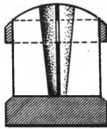
Пуля Ширинского-Шихматова. Первый образец.
