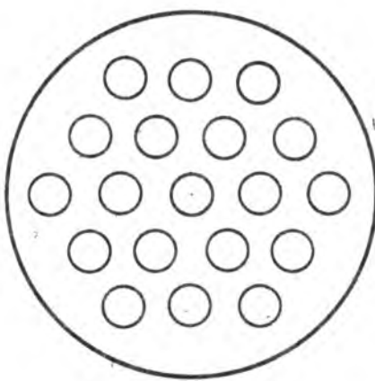
Картонная прокладка на порох с отверстиями диаметром 1,0—1,5 мм.
