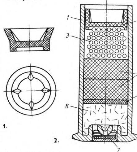
1. Пластмассовый дробовый пыж для металлической гильзы.
