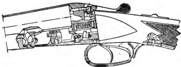
Устройство запирающего механизма ружья ИЖ-57.
