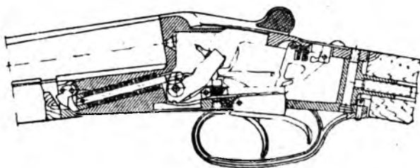
Устройство механизмов ружья ИЖ-58.
