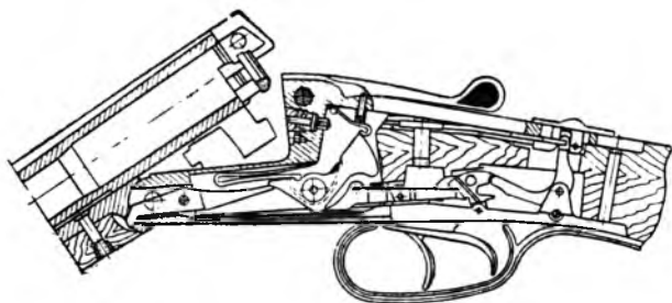
Устройство механизмов ружья ИЖ-54.
