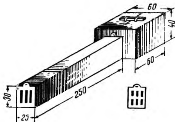
Учебная нора.
