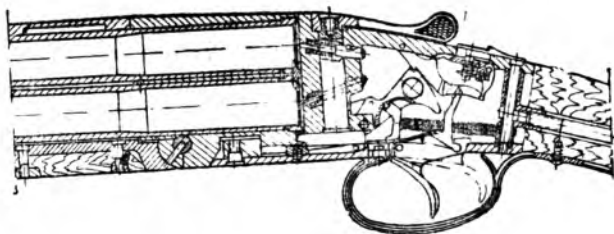
Устройство механизмов ружья ИЖ-59 «Спутник».
