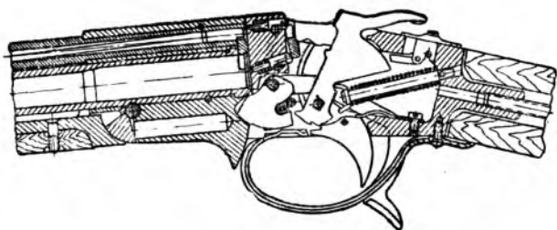
Устройство механизмов ружья ИЖ-56 «Белка».
