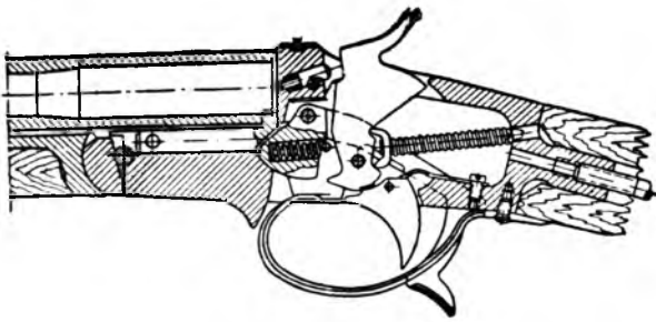
Устройство механизмов ружья ИЖК.
