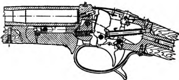
Устройство механизмов ружья ИЖКБ.
