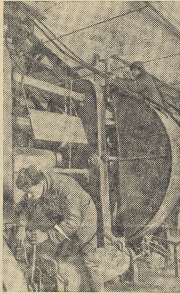
Монтируются машины и агрегаты в восстанавливаемом цехе ситцевобивной фабрики „Пролетарка“.
