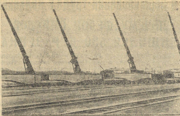
Батарея германских дальнбойных орудий типа „Верта“, установленных на железнодорожных платформах. Фото ТАСС.
