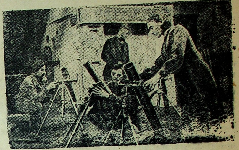
На снимке: Сборка минометов на Иском заводе. Справа налево: сборщики—слесари Н. Федорова, Н. Перов, Г. Шагин и Н. Сафронов. Они выполняют по две с половиной—три с половиной нормы. Фото В. Капустина
