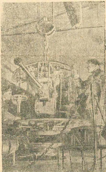
На Н-ском заводе. Боевой корабль скоро вступит в строй. На снимке: Установка автоматической пушки. Фото В. Тарасевича. Фотохроника ТАСС.
