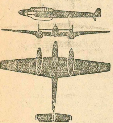
Немецкий истребитель Мессершмитт М-110. Вид сбоку, спереди и снизу.
