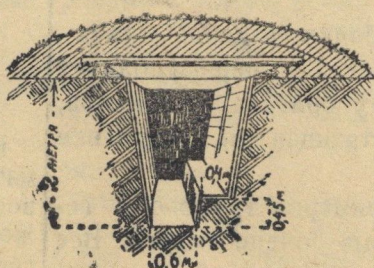
Рис. 2. Закрытая щель
