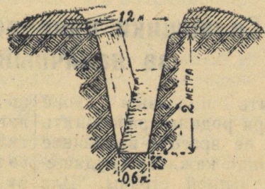
Рис. 1. Открытая щель.
