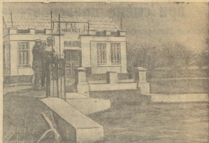
В прошлом году колхоз «Чекист» (Тимашевский район, Краснодарского края) своими средствами выстроил гидроэлектростанцию мощностью в 75 киловатт. В текущем году колхозники предполагают увеличить мощность станции вдвое.
