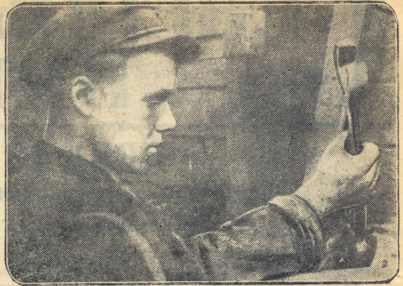
Слесарь-стахановец Череповецкого вагоноремонтного пункта В. М. Сорокин, выполняющий до двух с половиной норм, за ремонтом буферных стаканов. Фото Я. Кисина.
