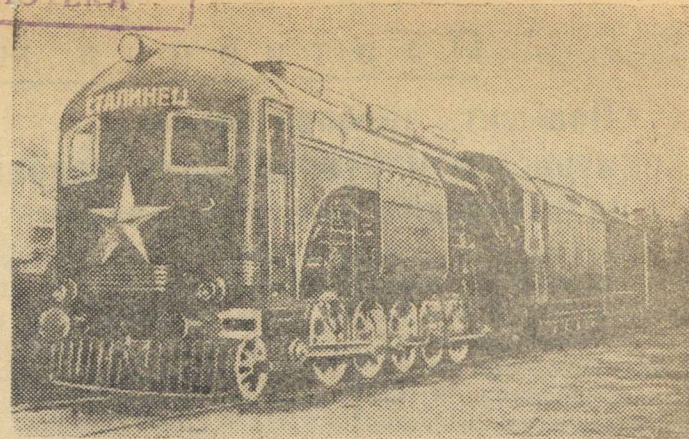
На снимке: первый советский товарный теплопаровоз „Сталинец“ с тендерконденсатором, имеющий комбинированный газопаровой двигатель, работающий на генераторном газе и паре. Построен Коломенским ордена Ленина машиностроительным заводом имени Куйбышева.
