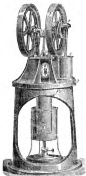
(Рис. 18). Моторъ для накачиванія воздуха въ акваріумъ, 45—110 р. по величинѣ.
