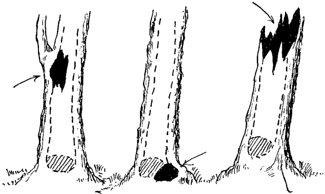
Типы берлог белогрудого медведя (по Г. Ф. Бромлею): слева направо — с верхним входом, приклеивая и в высоком пне; вход в убежище обозначен стрелкой, место лежки заштриховано
