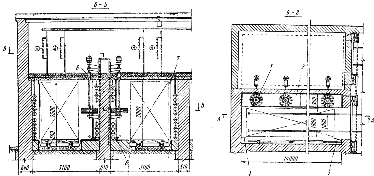
Рис. 19. Лесосушильная камера ВПКТИМ с осевыми реверсивными вентиляторами на вертикальных валах (Л. В. Сахновский и Б. С. Царев):
