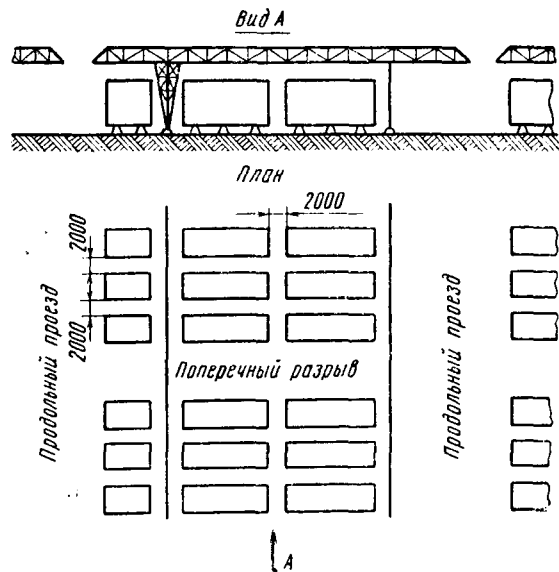
Рис. 94. Планировка склада для группы пакетных штабелей при укладке козловым краном
