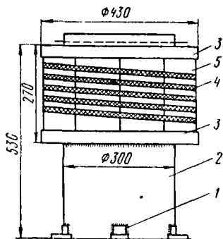
Рис. 120. Электрическая мангалка:
