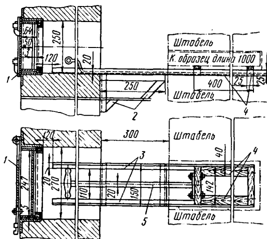
Рис. 122. Схема устройства приспособления для закладки образцов в камеры: 1 — дверка, 2 — кронштейн, 3 — направляющие, 4 — рамка, 5 — рукоятка
