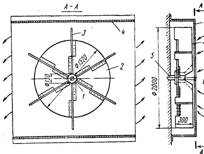
Рис. 45. Роторный вентилятор:
