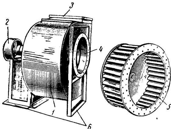
Рис. 44. Центробежный вентилятор:
