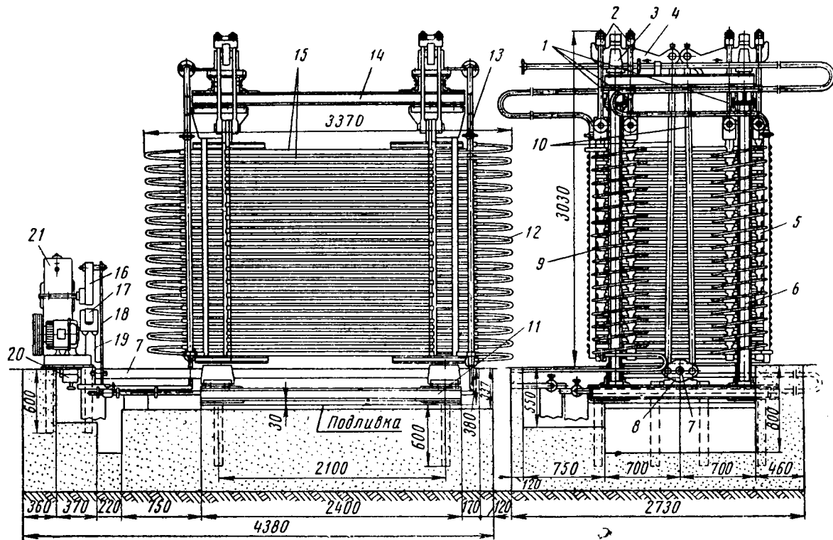
Рис. 108. Дыхательный пресс:
