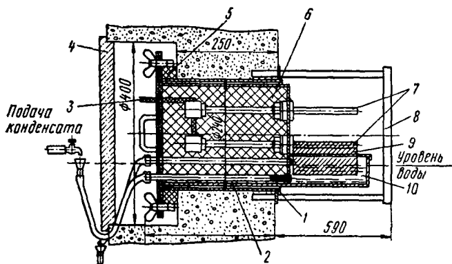
Рис. 62. Устройство для установки датчиков электропсихрометра в камере:
