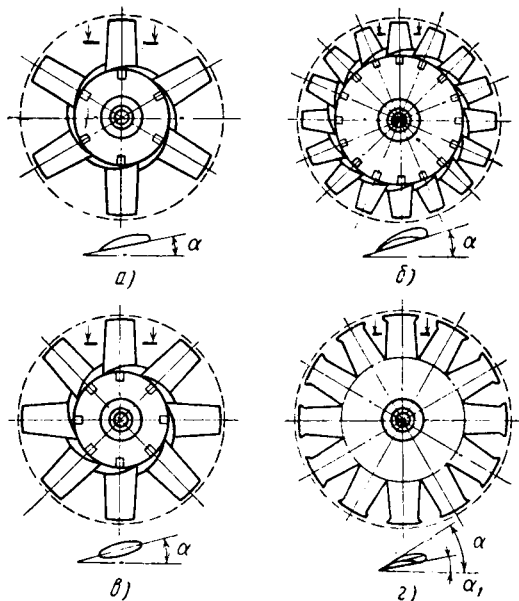
Рис. 48. Осевые вентиляторы ЦАГИ:
