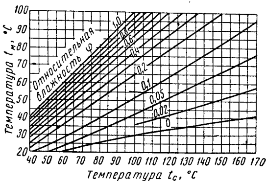
Рис. 1. Психрометрическая диаграмма
