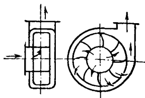
Рис. 47. Движение воздуха через центробежный вентилятор
