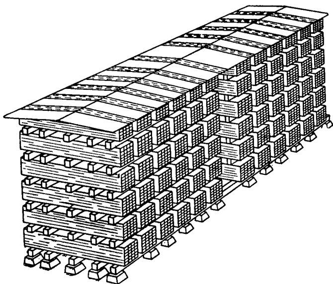
Рис. 92. Общий вид пакетного штабеля
