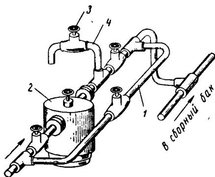
Рис. 40. Установка конденсатоотводчика:
