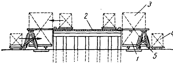
Рис. 66. Укладка штабелей с двух уровней:
