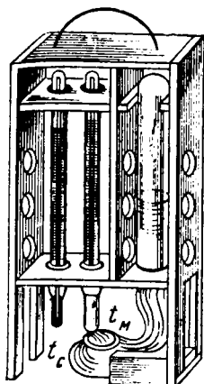
Рис. 55. Переносный психрометр
