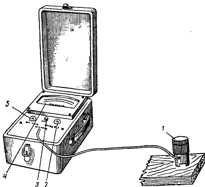
Рис. 7. Общий вид электровлагомера ЭВА-2М:
