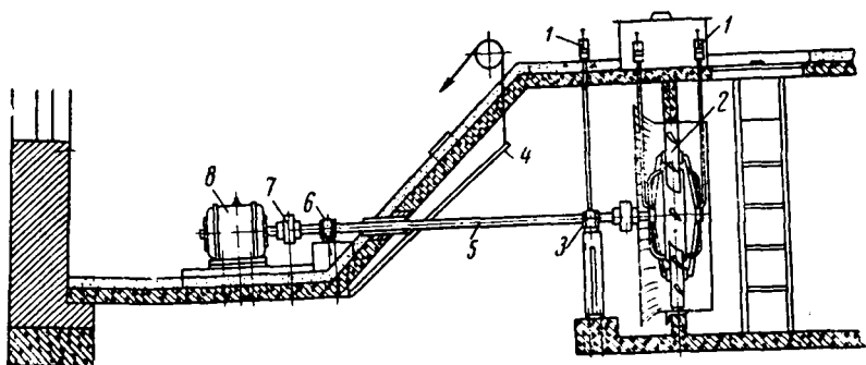
Рис. 49. Установка осевого вентилятора в сушильной камере непрерывного действия:
