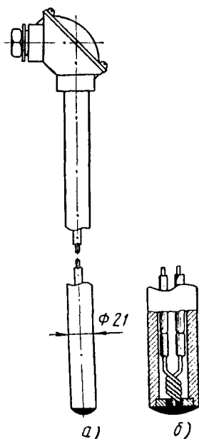
Рис. 60. Термопара ТХК-146:
