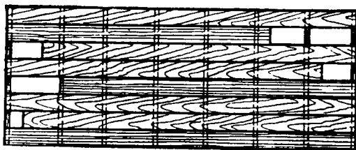
Рис. 82. Укладка в штабеля досок без шпаций разной длины вразбежку
