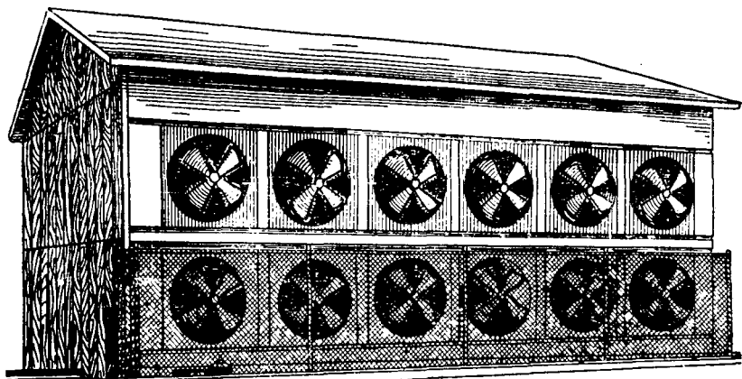
Рис. 106. Общий вид крытого сарая с продуванием штабелей атмосферным воздухом
