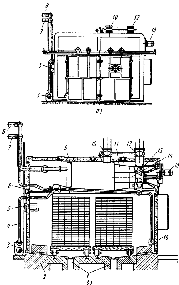
Рис. 26. Сборная металлическая камера Хильдебранд (ФРГ):
