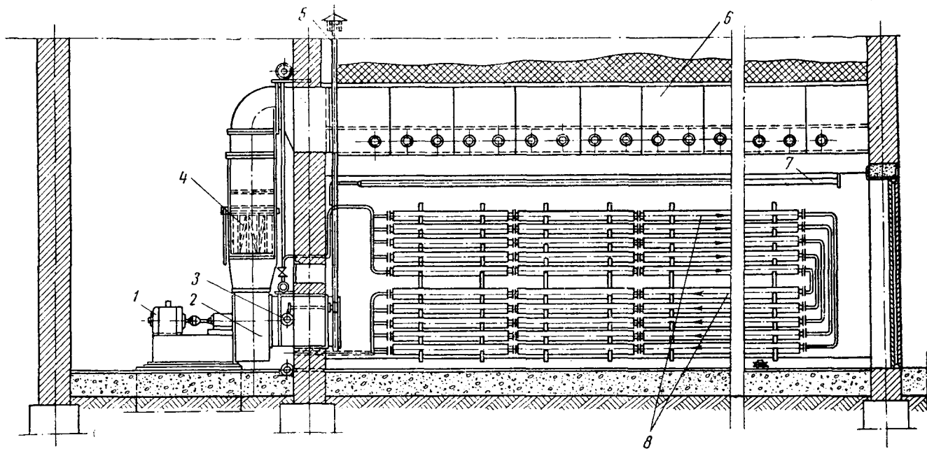
Рис. 21. Сушильная камера ВНИИДМАШ — Гидродревпром с эжекционной реверсивной циркуляцией: 1 — электродвигатель, 2 — центробежный вентилятор, 3 — патрубок с шибером для притока свежего воздуха, 4 — реверсивная коробка с перекидной заслонкой, 5 — вытяжная труба с шибером, 6 — распределительный воздухопровод с соплами, 7 — увлажнительная труба, 8 — calorifer
