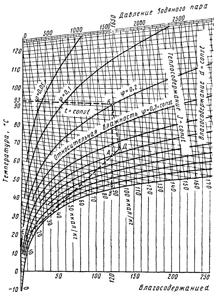
Рис. 2. I d -диаграмма влажного воздуха
