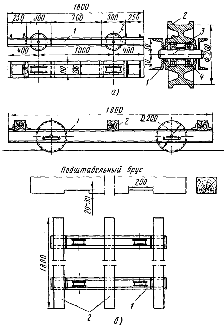
Рис. 75. Устройство трека и треновой тележки:
