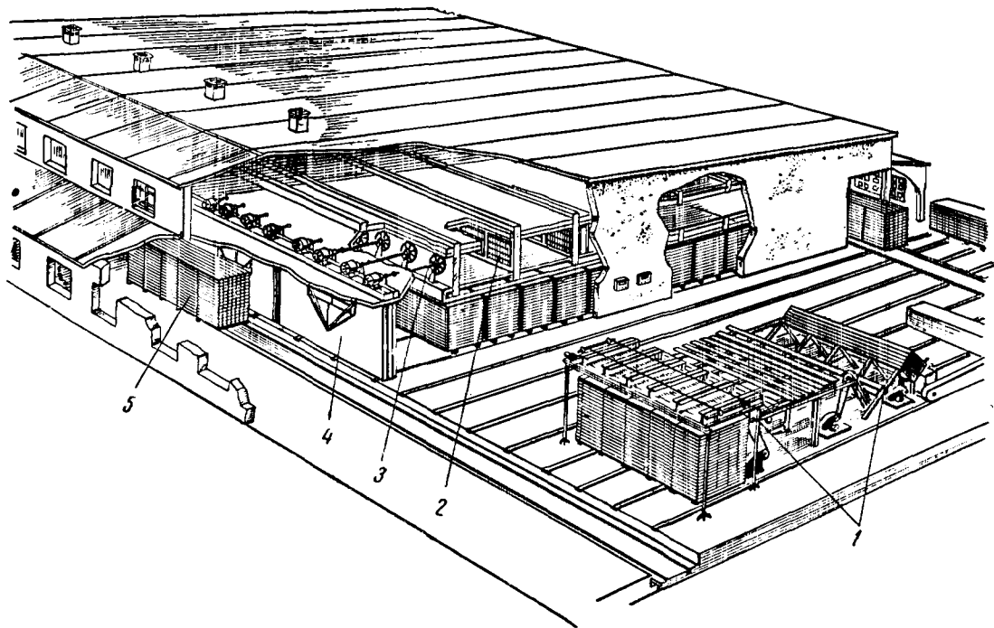
Рис. 28. Сушильные камеры непрерывного действия ЦНИИМОД-49 с противоточной прямолинейной циркуляцией и поперечной загрузкой штабелей: 1 — штабелеукладчик, 2 — пластинчатые calorиферы, 3 — осевые вентиляторы с электродвигателями, 4 — загрузочные двери, 5 — штабель
