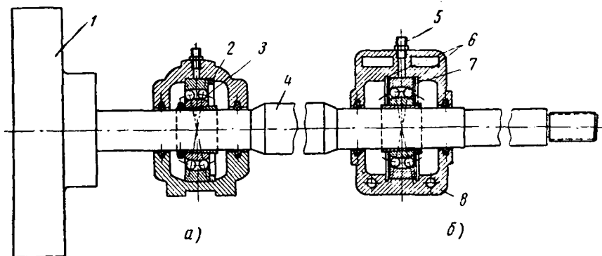
Рис. 50. Подшипники вентиляторного вала:
