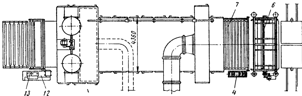
Рис. 111. Газовая роликовая сушилка СРГ-25:
