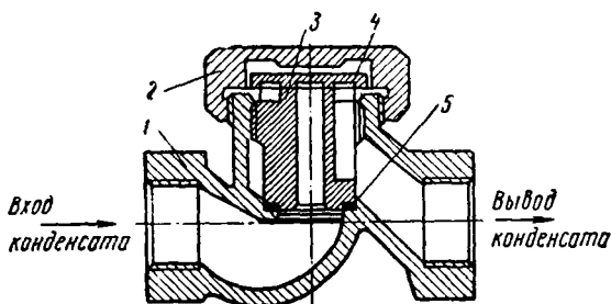
Рис. 41. Конденсатоотводчик термодинамический 45ч12нж:
