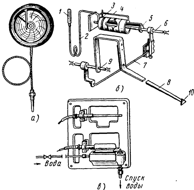
Рис. 58. Манометрический термометр:
