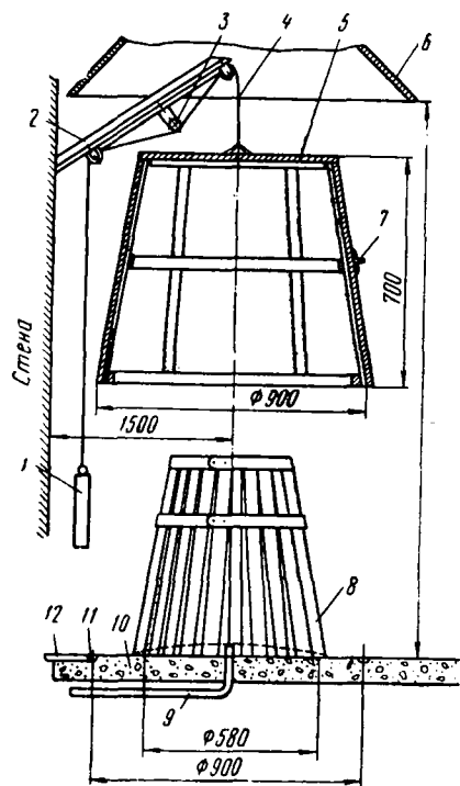
Рис. 117. Парный колпак для пропарки бочечных остовов:
