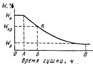
Рис. 9. График процесса сушки древесины
