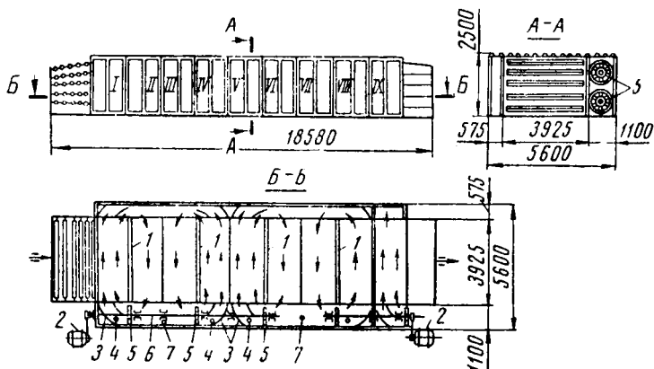
Рис. 110. Схема паровой сушилки СРГ-4 с поперечной циркуляцией:
