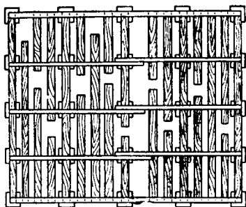
Рис. 97. Штабель пиломатериалов с расположением крайних прокладок (реек) заподлицо с торцами досок и брусков
