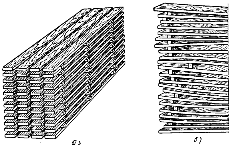
Рис. 96. Правильно (а) и неправильно (б) уложенный пакет
