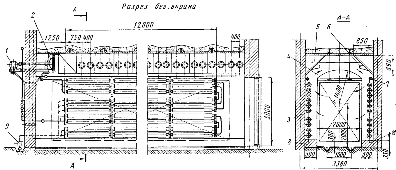
Рис. 20. Сушильная камера ЦНИИМОД — Гипродрев с эжекционной реверсивной циркуляцией (И. В. Кречетов): 1 — электродвигатель, 2 — осевой высоконапорный вентилятор, 3 — calorifer, 4 — подвесной экран, 5 — нагнетательный распределительный воздуховод с соплами, 6 — сопла, 7 — увлажнительная труба, 8 — экран, 9 — конденсатоотводчик
