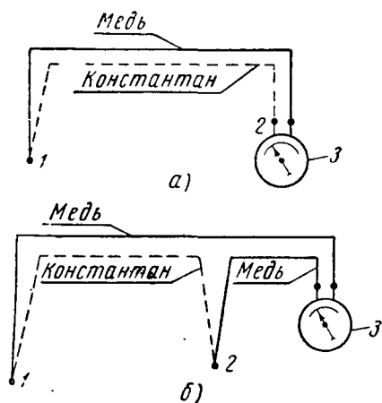
Рис. 59. Схемы термопар:
