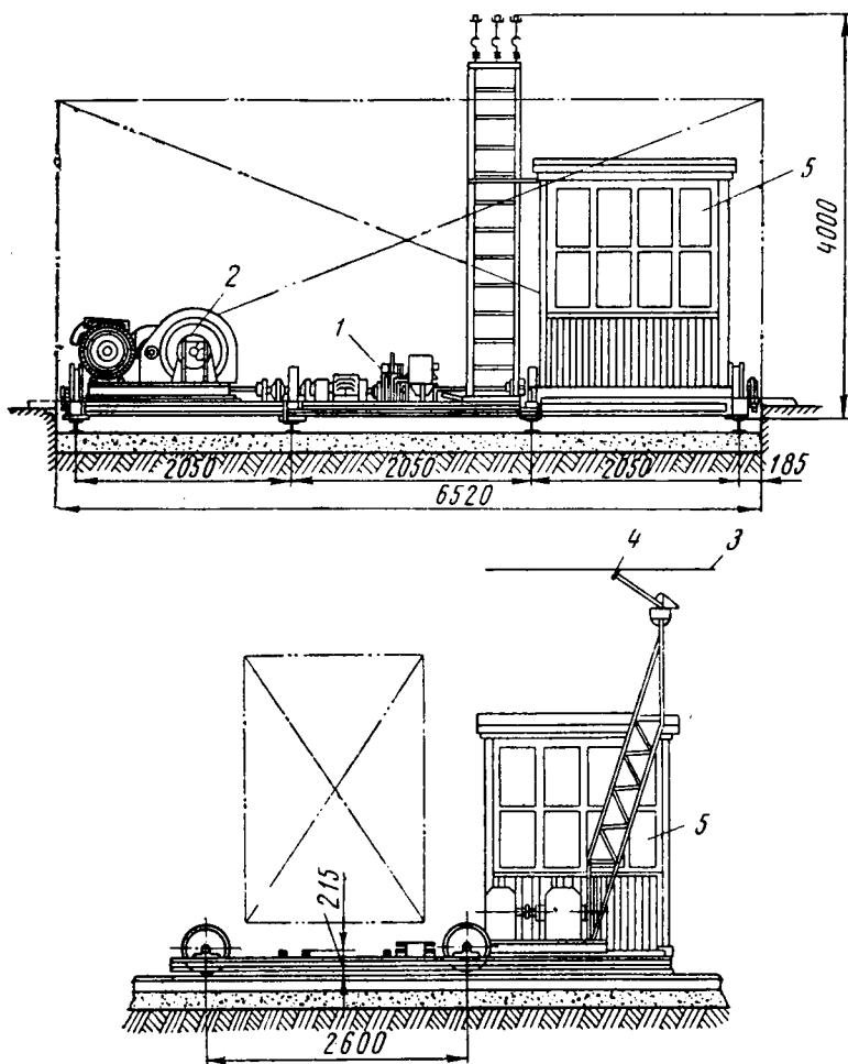
Рис. 76. Траверсная электрифицированная тележка ЭТ-20:
