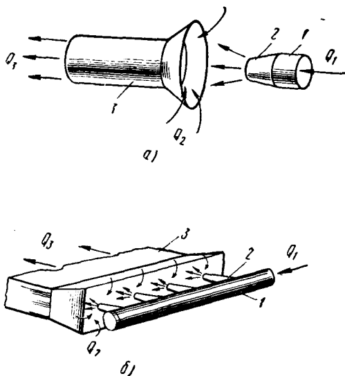
Рис. 51. Схема действия эжектора: а — с круглым каналом, б — с прямоугольным каналом; 1 — воздуховод, 2 — насадки, 3 — смешивательный канал
