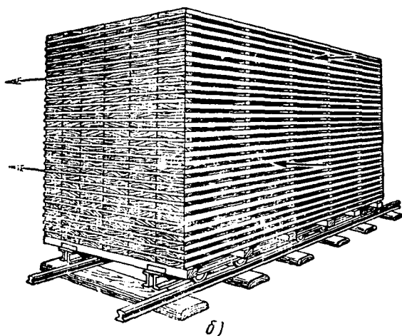
Рис. 84. Способы укладки пиломатериалов в штабеля в зависимости от направления движения сушильного агента:
