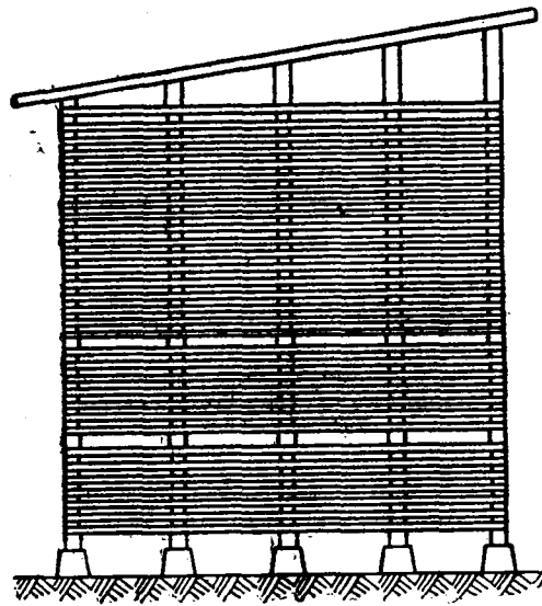
Рис. 100. Расположение горизонтальных каналов по высоте штабеля
