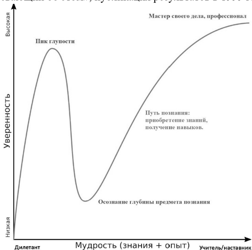
Рисунок 67. Кривая Даннинга–Крюгера.
