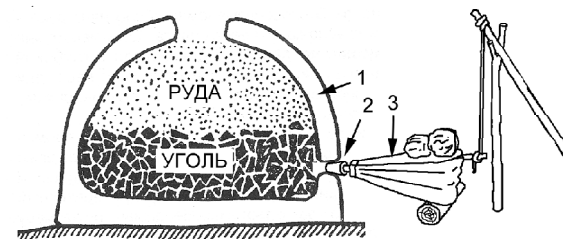
Рис. 4. Разрез сыродутного горна:
