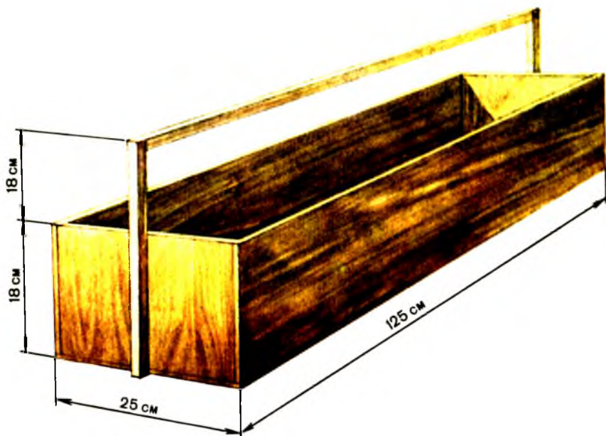
Р и с. 3 Поилка для гусят старших возрастов
