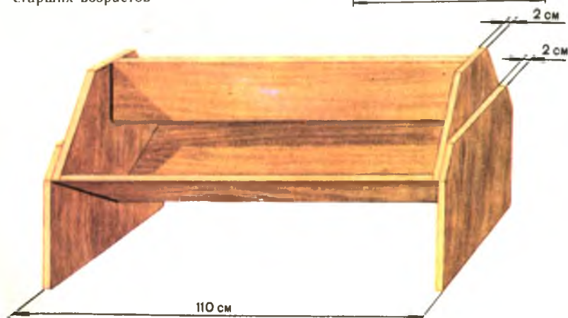
Р и с. 5 Кормушка для гусят старших возрастов
