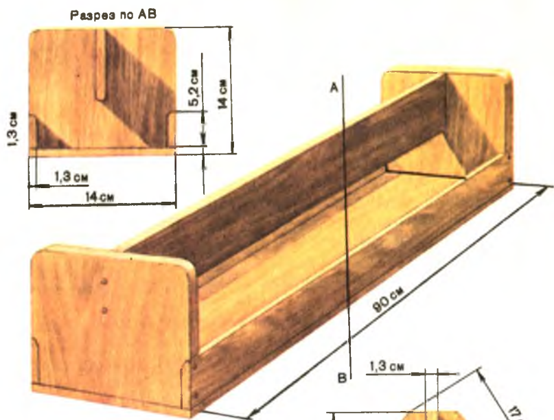
Р и с. 4 Кормушка для гусят до 15-дневного возраста
