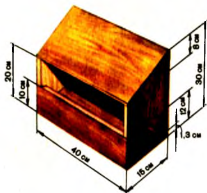
Рис. 1 Кормушка для минеральных кормов
