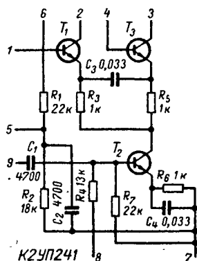
Рис. 18. Принципиальная схема К2УП241.
