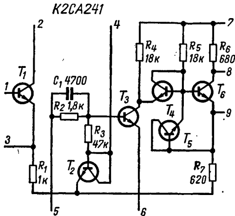
Рис. 21. Принципиальная схема К2СА241.
