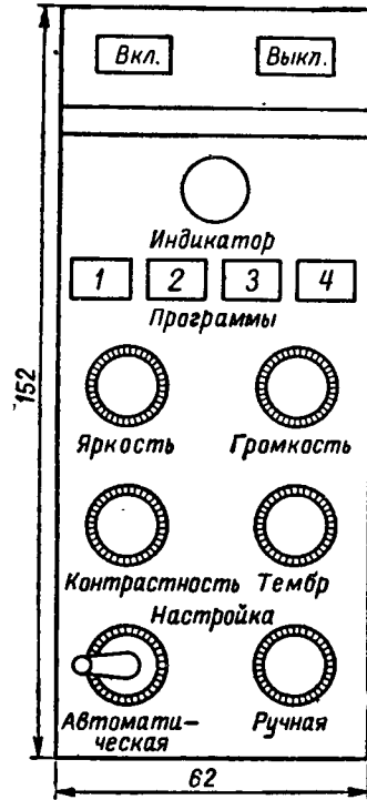
Рис. 2. Расположение органов управления на лицевой панели телевизора.
