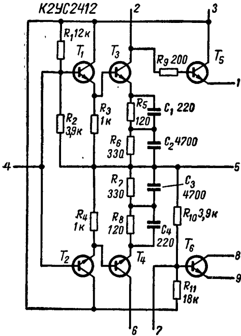
Рис. 26. Принципиальная схема K2YC2412.
