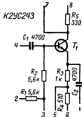
Рис. 4. Принципиальная схема К2УС243.
