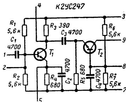
Рис. 8. Принципиальная схема К2УС247.
