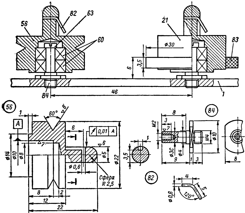
Рис. 11. Приемный и подающий узлы.
