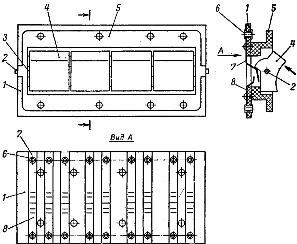
Рис. 10. Устройство регистрового переключателя ( B_{37} , B_{38} , B_{43} , B_{44} ).
