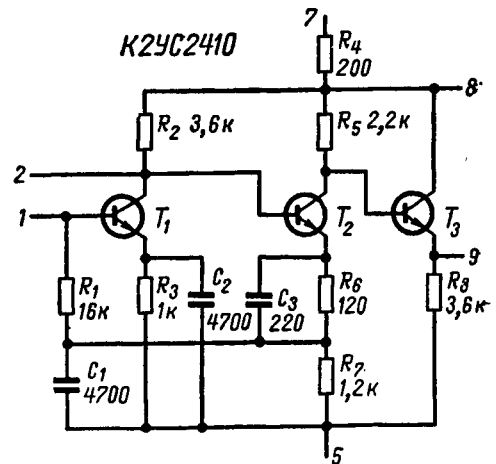
Рис. 24. Принципиальная схема К2УС2410.
