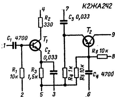
Рис. 12. Принципиальная схема К2ЖА242.
