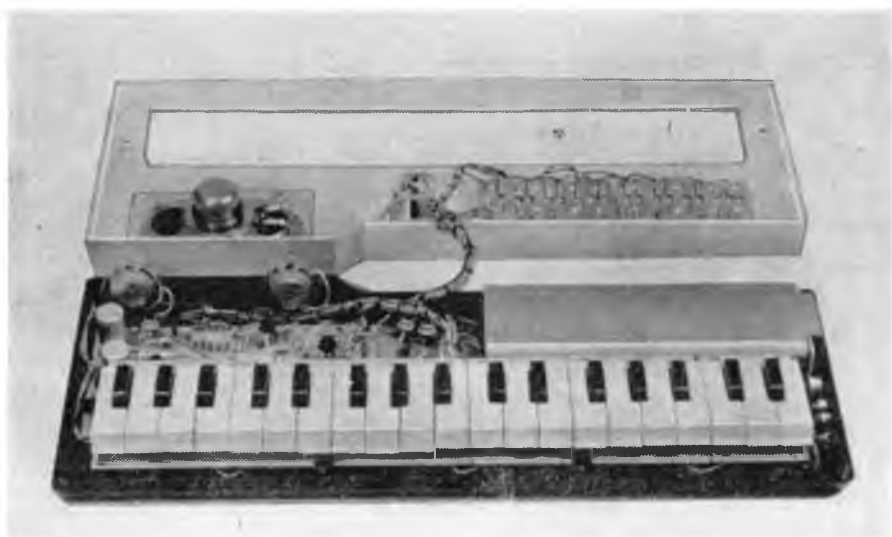
Рис. 5. Размещение деталей в корпусе инструмента.
