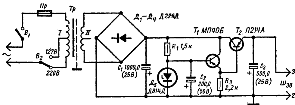
Рис. 2. Принципиальная схема сетевой приставки-выпрямителя.
