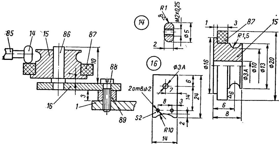
Рис. 12. Узел обрезиненного ролика
