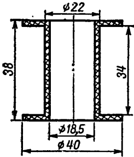
Рис. 4. Каркас катушки выходного трансформатора строк.
