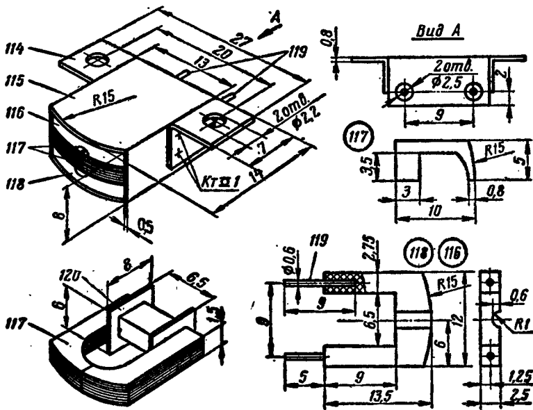
Рис. 18. Универсальная головка.
