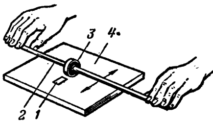
Рис. 19. Изготовление прокладки рабочего зазора универсальной головки.
