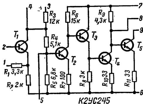
Рис. 6. Принципиальная схема К2УС245.
