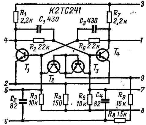
Рис. 29. Принципиальная схема K2TC241.
