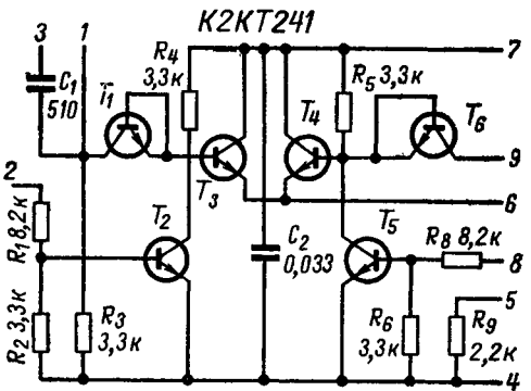
Рис. 30. Принципиальная схема K2KT241.
