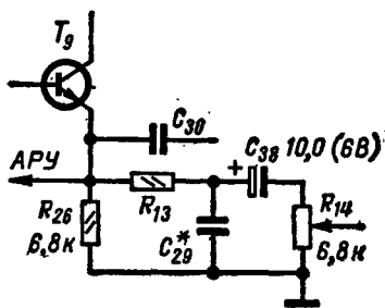
Рис. 2. Изменения в схеме детектора для устранения помех при регулировке громкости.
