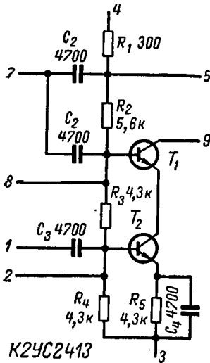
Рис. 27. Принципиальная схема K2YC2413.
