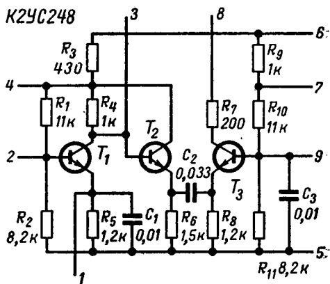
Рис. 9. Принципиальная схема К2УС248.
