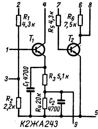
Рис. 13. Принципиальная схема К2ЖА243.
