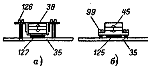
Рис. 22. Установка универсальной (а) и стирающей (б) головок на планке блока головок.
