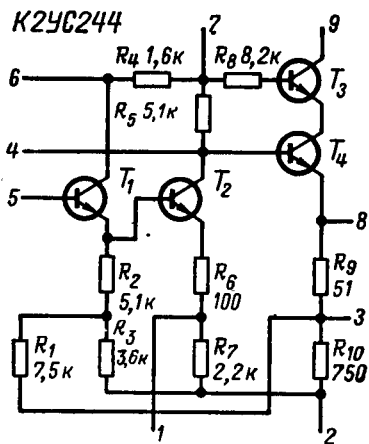
Рис. 5. Принципиальная схема К2УС244.
