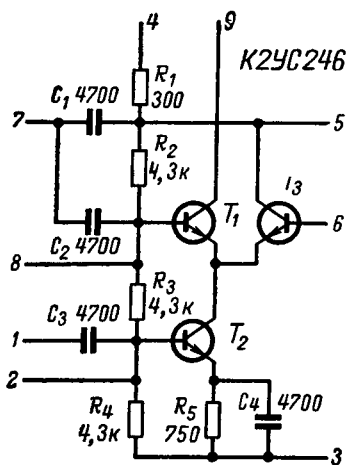
Рис. 7. Принципиальная схема К2УС246.
