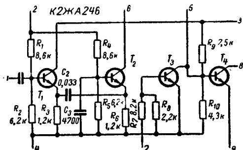
Рис. 16. Принципиальная схема К2ЖА246.
