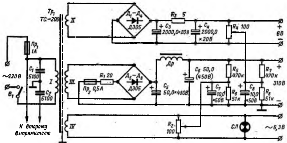
Рис. 3. Принципиальная схема блока питания.
