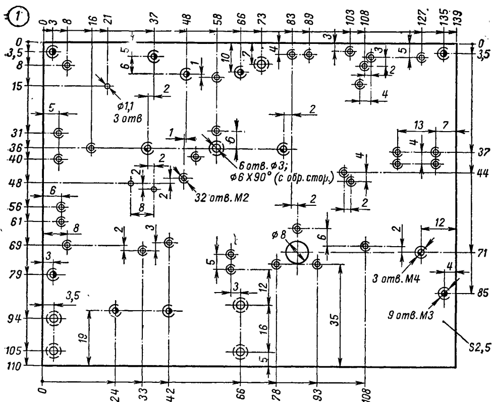
Рис. 7. Панель лентопротяжного механизма, Д16А-Т.
