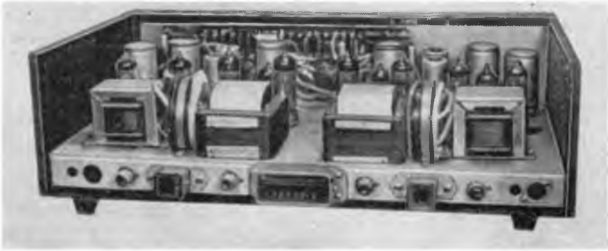
Рис. 5. Вид на монтаж усилителей блока.
