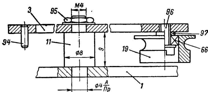
Рис. 14. Узел привода приемного узла.
