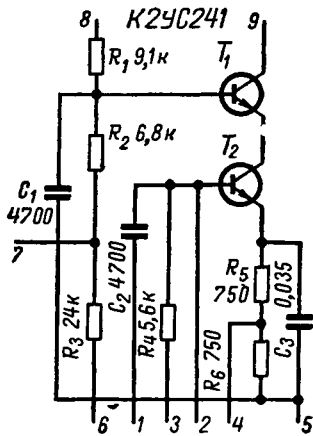
Рис. 2. Принципиальная схема К2УС241.
