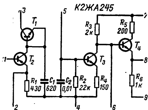
Рис. 15. Принципиальная схема К2ЖА245.
