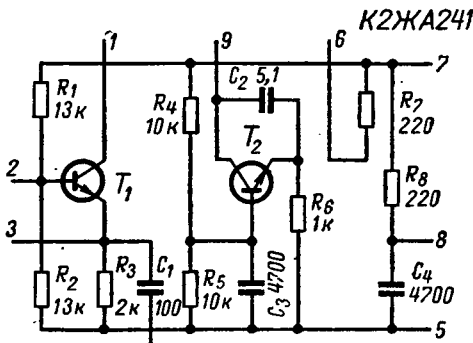
Рис. 11. Принципиальная схема К2ЖА241.
