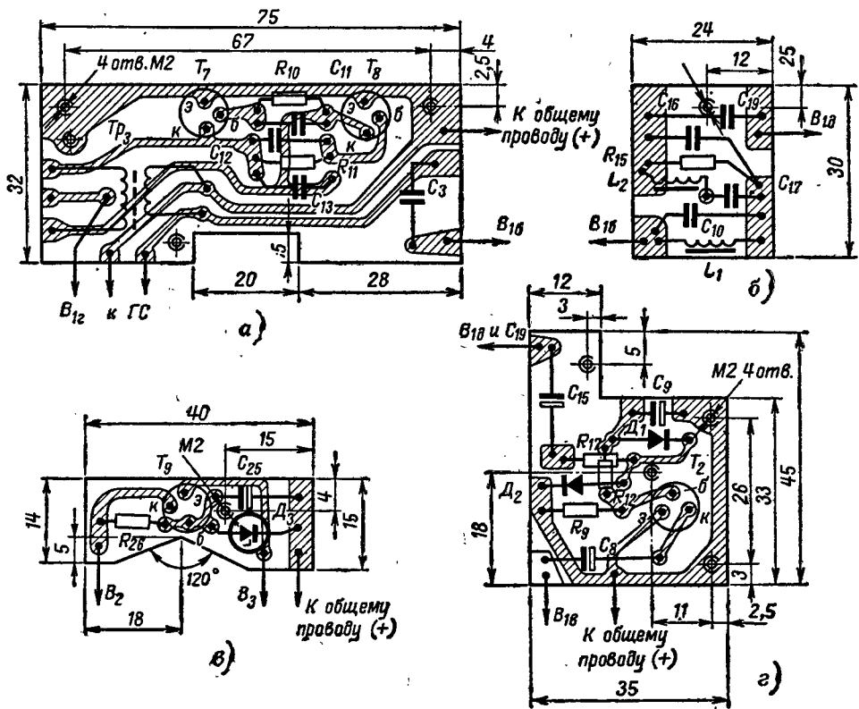
Рис. 4. Печатные платы и схемы соединений.
