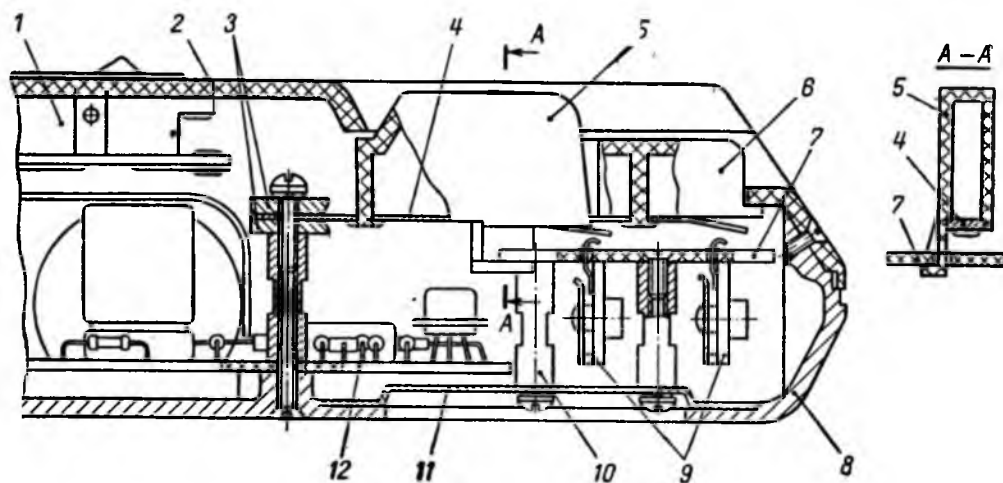
Рис. 6. Устройство клавиатуры.
