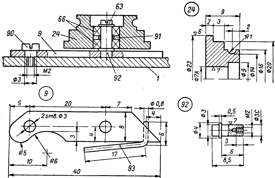
Рис. 13. Узел промежуточного ролика.
