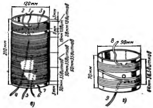
Радиоприемник С. И. Шапошникова.
