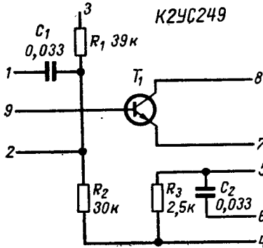
Рис. 10. Принципиальная схема К2УС249
