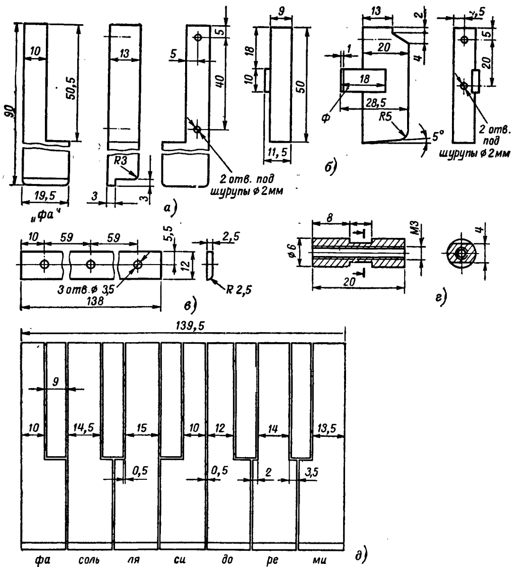
Рис. 8. Детали клавиатуры.
