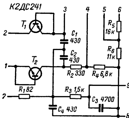
Рис. 19. Принципиальная схема К2ДС241.
