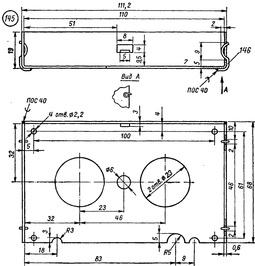
Рис. 24. Подкассетник.
