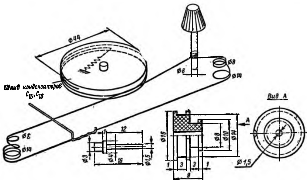
Рис. 5. Кинематическая схема и детали шкально-верньерного механизма.
