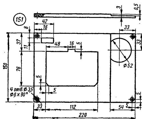
Рис. 27. Верхняя панель магнитофона (декоративная пластмасса).
