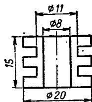
Рис. 3. Радиатор транзистора T_{212} .
