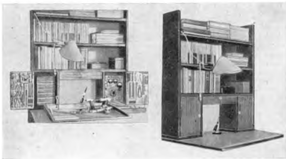
Рабочее место радиолюбителя.
