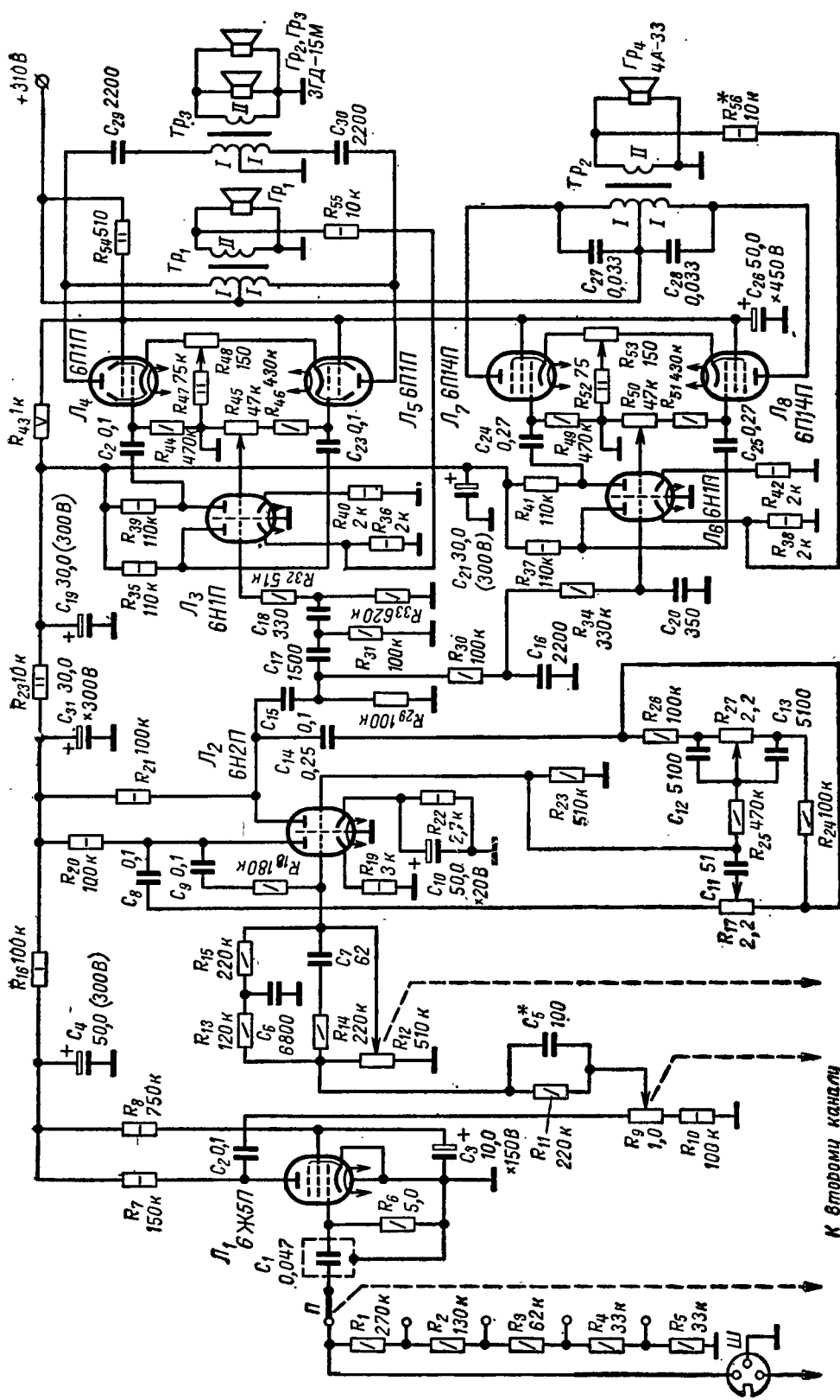
Рис. 2. Принципиальная схема усилителя.
