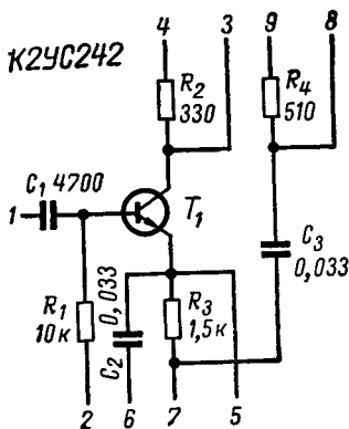
Рис. 3. Принципиальная схема К2УС242.
