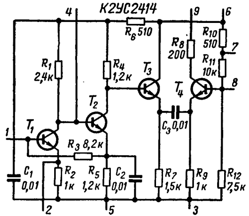
Рис. 28. Принципиальная схема K2YC2414.
