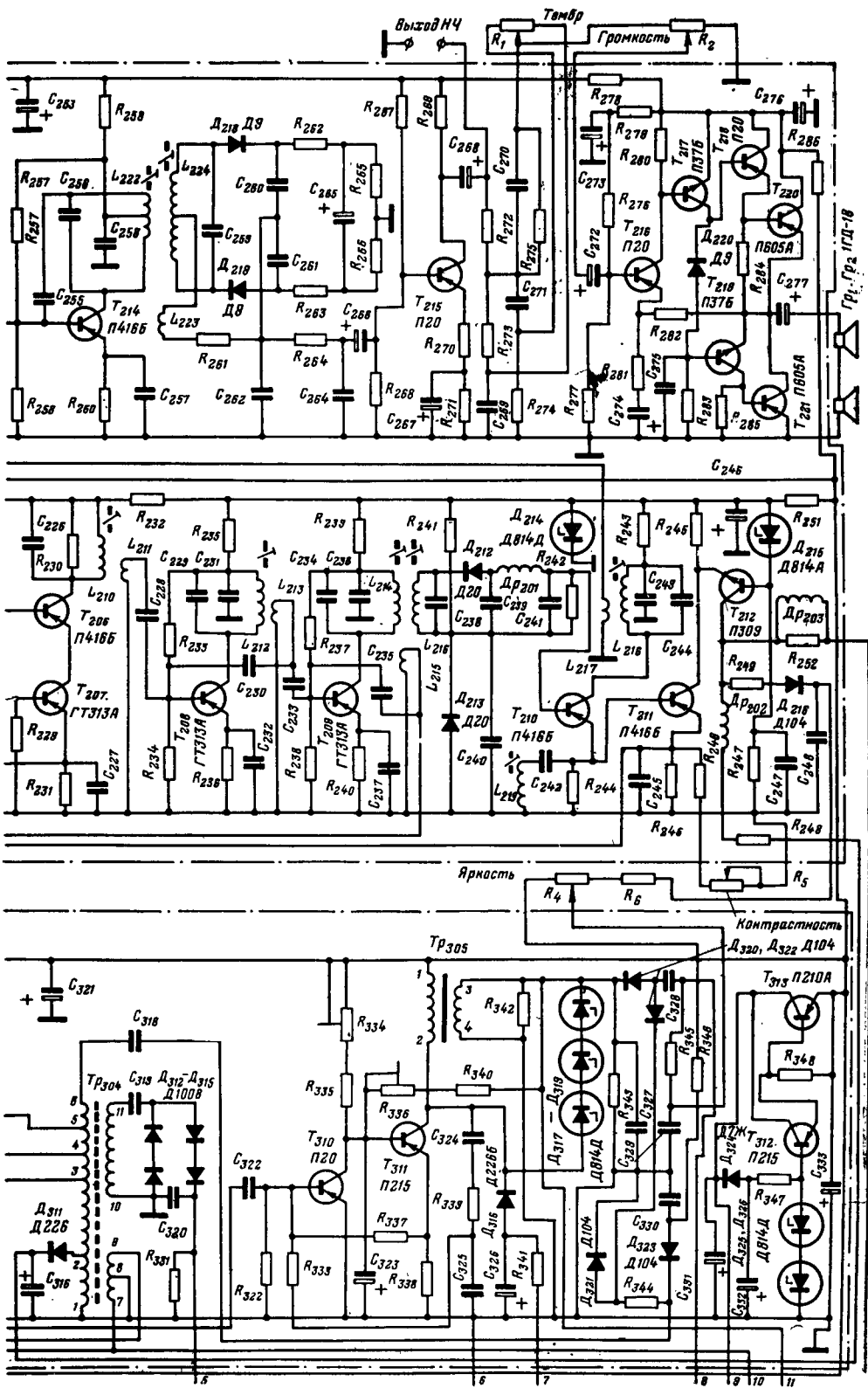
схема телевизора.
