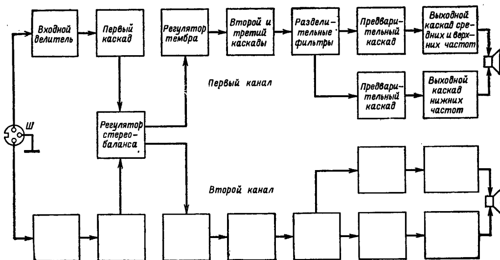
Рис. 1. Структурная схема усилителя.
