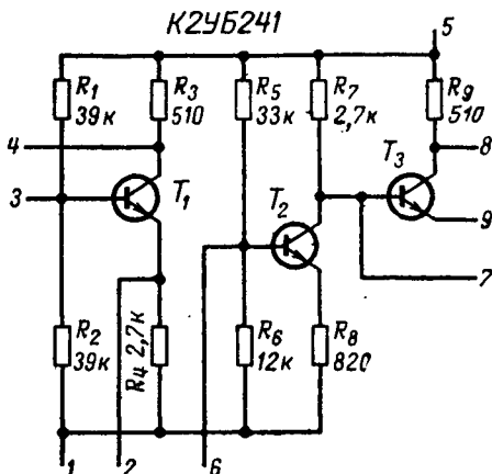
Рис. 22. Принципиальная схема К2УБ241.
