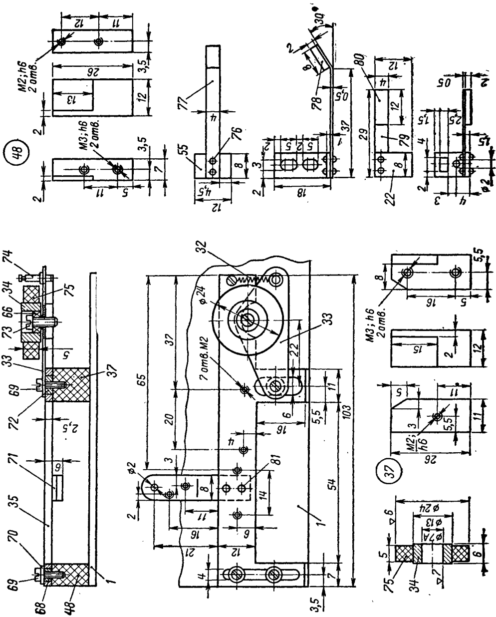
Рис. 10. Узел прижимного ролика и подтормаживающего устройства. 1 — панель ЛПМ; 22 — угольник-кронштейн Ст.10кп; 32 — пружина, проволока стальная класса 1 с диаметром 0,5 мм; 33 — рычаг, Л162-Т; 34 — втулка Л1С59-1; 35 — планка блока головок Д16А-Т; 37, 48 — стойки блока головок Фторопласт; 55 — угольник-кронштейн Ст.10кп; 66 — шариковый подшипник 2000083, запрессовать в деталь 34; 68 — кольцо, Л1С59-1, 2 шт.; 69 — винт М2Х8, 3 шт.; 70 — шайба, 2 шт.; 71 — планка, Д16А-Т, соединить с деталью 36 закладками 81 (после клееки спилить заподлицо); 72 — кольцо, Л1С59-1; 73 — винт М2Х6; 74 — стойка, Ст.45, расклепать в детали 33; 75 — кольцо резинового, приклеить к детали 34 клеем 88-н; 76 — заклепка Ø 1X3, 4 шт.; 77 — пружина подтормаживающего устройства подающего узла, Бр ОФ6,5Х0,15, соединить с деталью 55 двумя закладками 76; 78 — накладка, фетр, приклеить к детали 77 клеем 88-н; 79 — пружина подтормаживающего устройства приемного узла, Бр.СФ6,5Х0,15, соединить с деталью 22 двумя закладками 76; 80 — накладка, фетр, приклеить к детали 79 клеем 88-н; 81 — заклепка Ø 1,5Х6, 2 шт.
