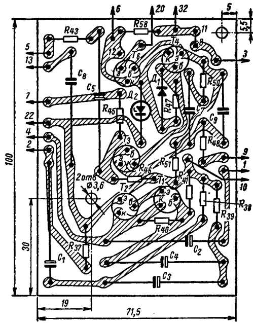
Рис. 3. Печатная плата и схема соединительного генератора тона, буферного каскада и генератора вибрато.
