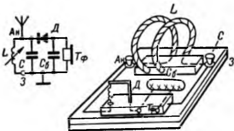
Радиоприемник Оганова.
