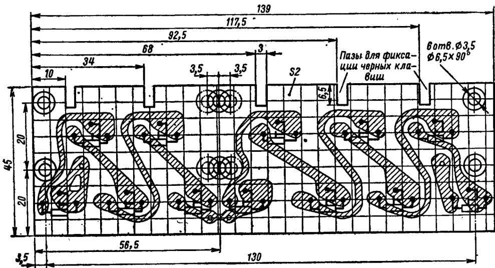
Рис. 9. Печатная плата и схема соединений подстроечных резисторов.
