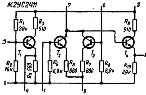
Рис. 25. Принципиальная схема K2YC2411.
