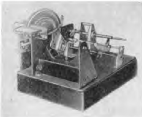
Намоточный станок (использованы детали трофейной радиостанции).
