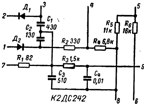
Рис. 20. Принципиальная схема К2ДС242.
