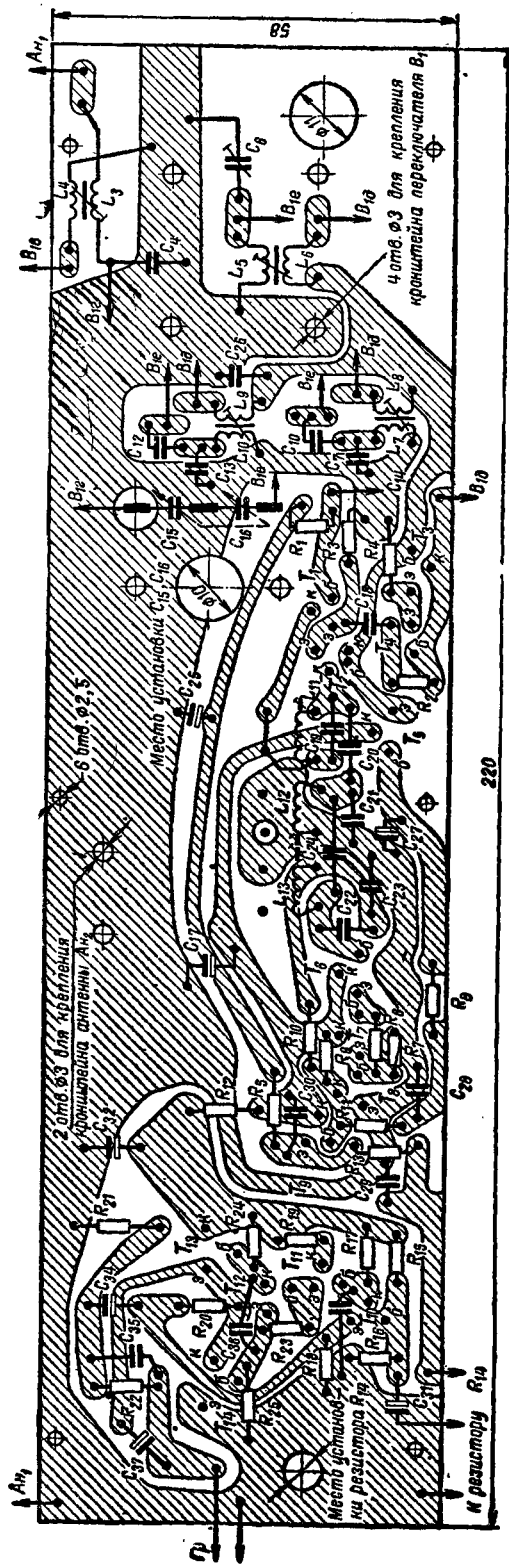
Рис. 3. Печатная плата и схема соединения приемника. Конденсаторы C_{3z} , C_{36} и резистор R_{25} при налаживании устанавливаются со стороны печатных проводников.
