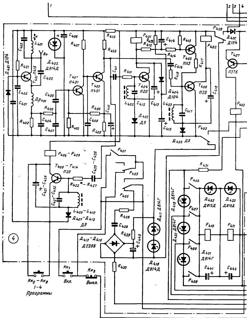
Принципиальная схема телевизора
