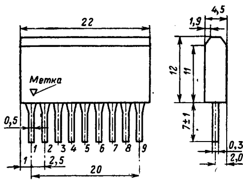
Рис. 1. Габаритный чертеж микросхемы серии К224.
