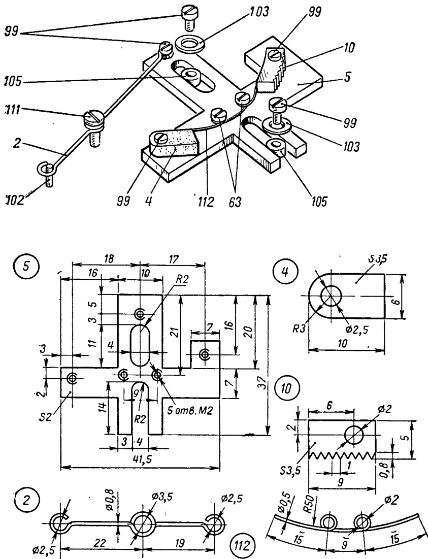
Рис. 16. Тормозное устройство.
