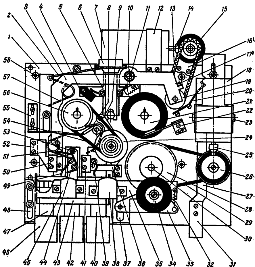
Рис. 6. Сборочный чертеж лентопротяжного механизма.
