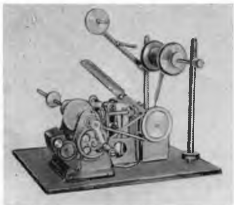
Намоточный станок.
