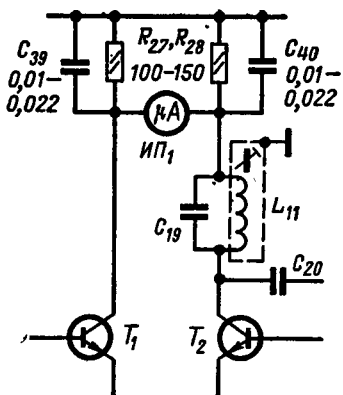
Рис. 7. Принципиальная схема смесителя со стрелочным индикатором настройки.
