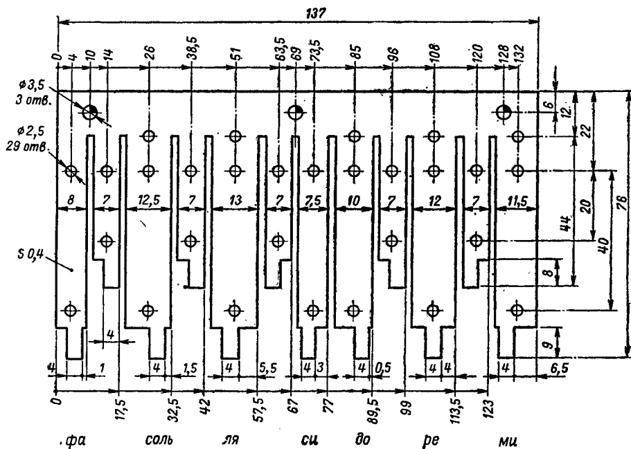
Рис. 7. Контактная гребенка, бронза.
