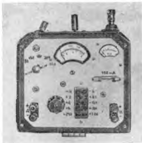
Стенд для испытания переносных радиостанций.
