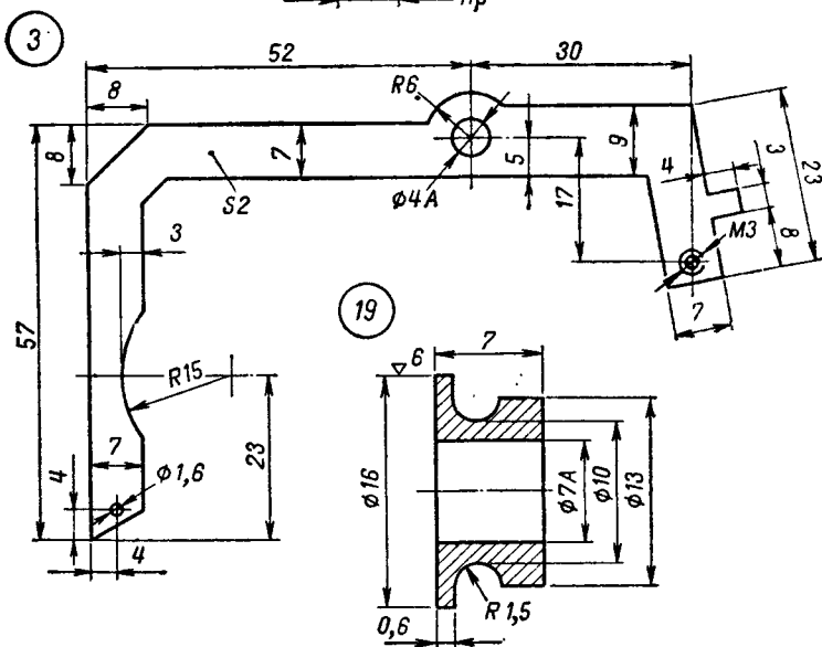
Рис. 15. Переключатель рода работ.
