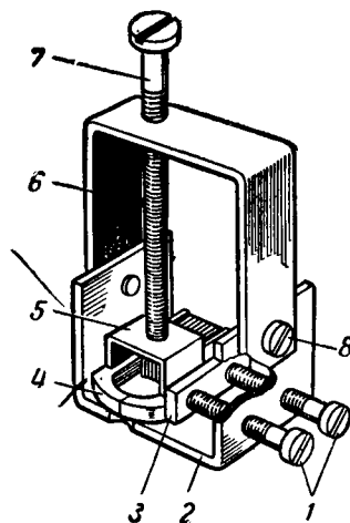
Рис. 20. Приспособление для сборки универсальной головки.
