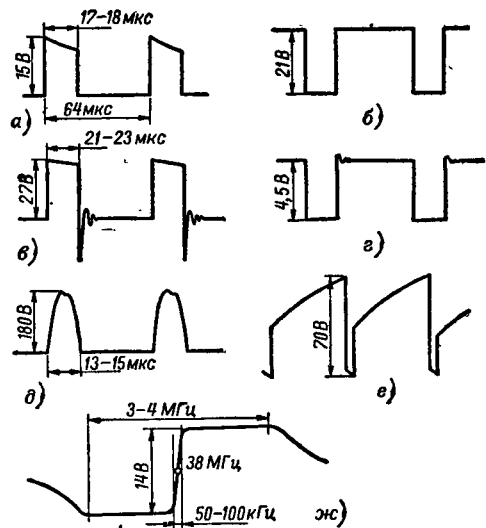
Рис. 5. Осциллограммы напряжений.
