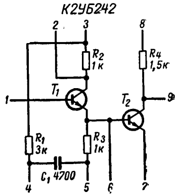
Рис. 23. Принципиальная схема К2УБ242:
