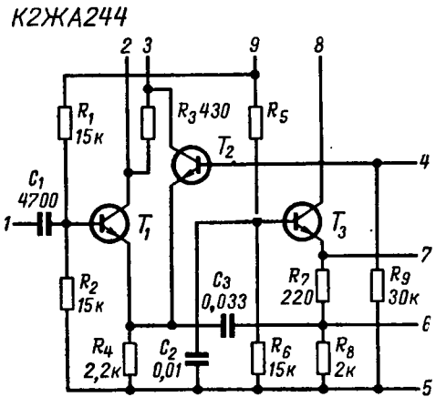
Рис. 14. Принципиальная схема К2ЖА244.
