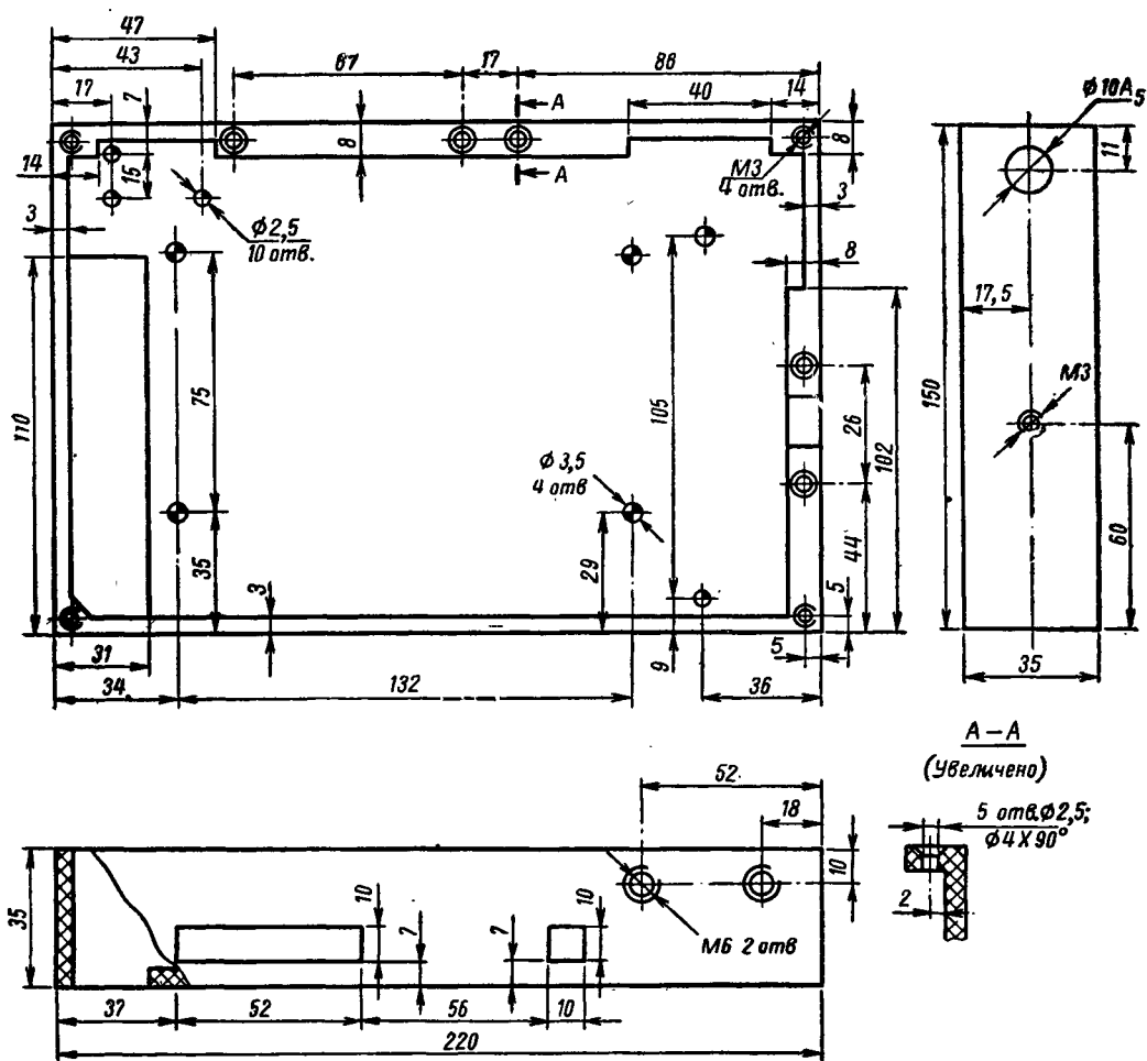
Рис. 26. Корпус магнитофона (полистирол).
