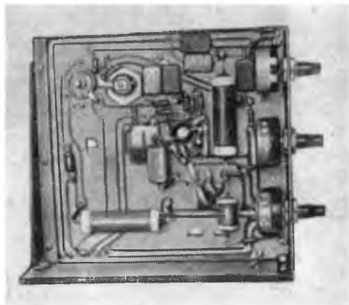
Самодельная печатная плата строчной раз- вертки телевизора.
