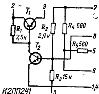
Рис. 17. Принципиальная схема К2ПП241.
