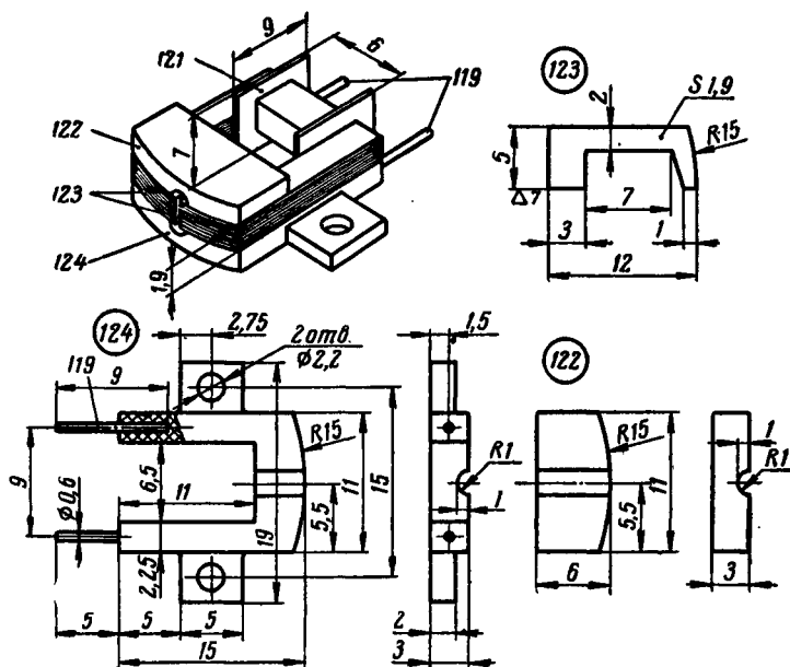
Рис. 21. Стирающая головка.
