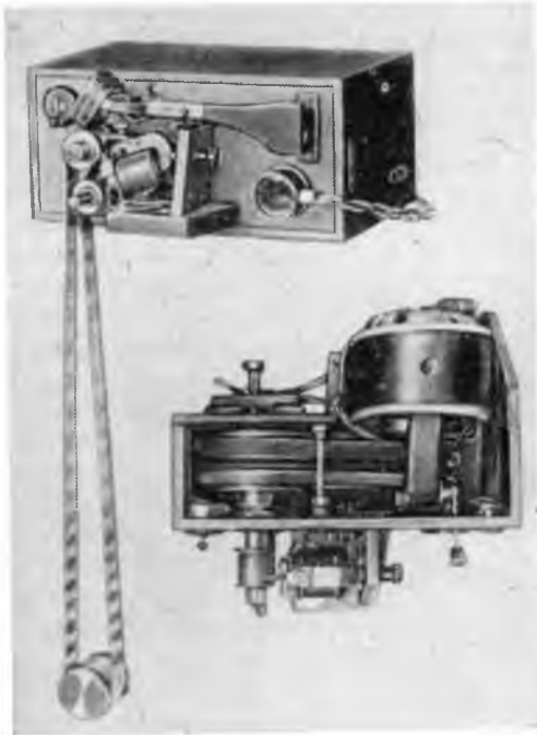
Звукозаписывающий аппарат.
