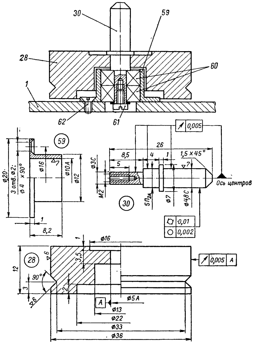
Рис. 8. Узел ведущего вала.
