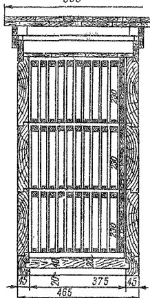
Поперечный разрез 550
