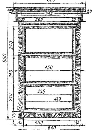
Продольный разрез 625
