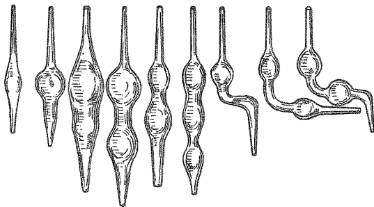
Рис. 5. Модели пипеток.
