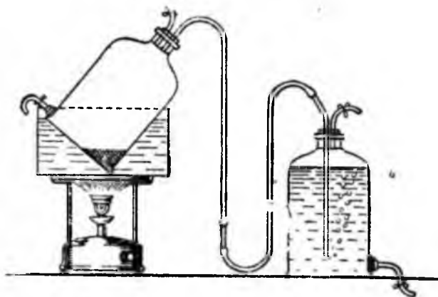
Рис. 41. Расположение бутылей для приготовления хлорацита по Шауфлеру.
