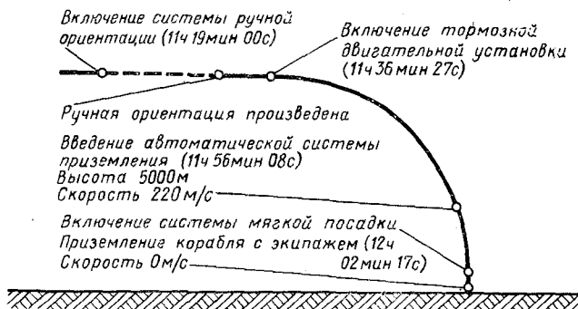
Схема спуска корабля «Восход-2». Время указано московское
