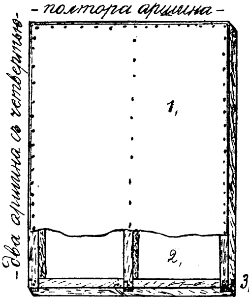
Рис. 3. Полотняная парниковая рама для позднихъ парниковъ, устроенныхъ въ первыхъ числахъ апрѣля мѣсяца. 1, Натянутый бѣлый коленикъ или полотно и прибитъ обойными гвоздями; 2, часть рамы открыта съ той цѣлью, чтобы можно было видѣть устройство самой рамы; 3, скрѣпленіе угловъ рамы.
