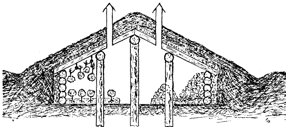
Рис. 19. Поперечный разрѣзъ овощного подвала съ конца. Въ боковыхъ внутреннихъ помѣщеніяхъ подвала: на лѣво—посаженные и подвѣшенные кочны б. к. капусты; на право—сложенные въ кучи корни овощныхъ растений.
