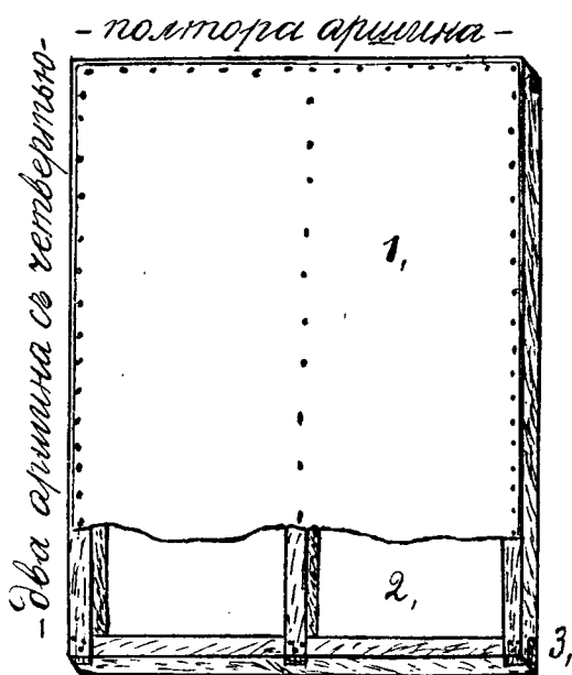
Рис. 3 Полотнянная парниковая рама для капустныхъ парниковъ, устроенныхъ въ первыхъ числахъ апрѣля мѣсяца. 1, Натянутый коленкоръ или полотно и прибитъ обойными гвоздями; 2, часть рамы открыта съ той цѣлью, чтобы можно было видѣть устройство самой рамы; 3, скрѣпленіе угловъ рамы.
