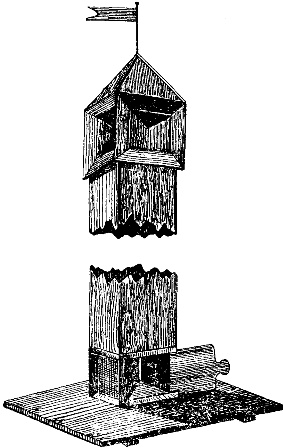
Рис. 1. Внѣшній видъ трубы системы Муира для вентиляціи.
