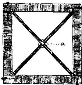
Рис. 2. Поперечный разрѣзъ трубы системы Муира.
