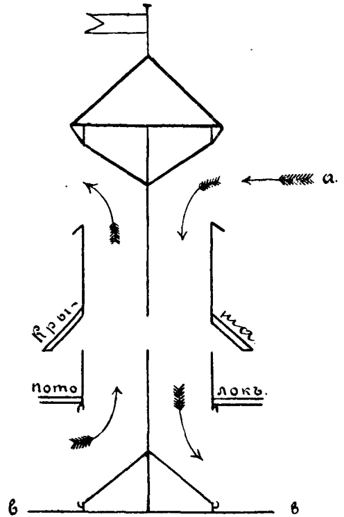
Рис. 3. Схематическій рисунокъ вертикальнаго разрѣза трубы системы Муира, показывающій входъ свѣжаго и выходъ испорченнаго воздуха.
