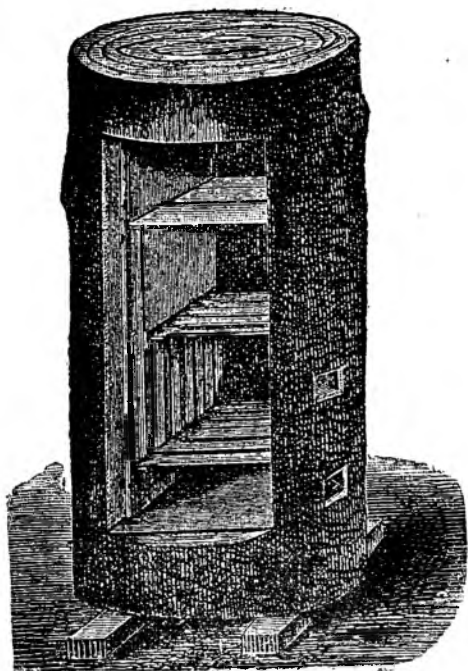
Рис. 275. Улучшенная рамочная колода.
