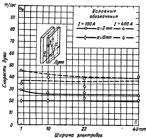
Рис. 3. Зависимость скорости движения дуги от ширины электродов при H = 200 \text{ Oe} .
