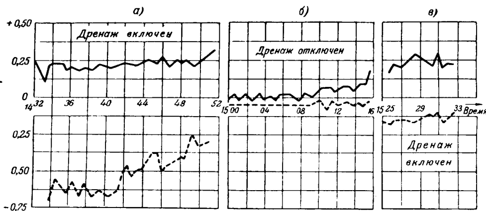
Рис. 2. Влияние дренажа кабелей АТС на потенциалы (в В) трубопровода; по оси абсцисс отложено время (часы и минуты)
