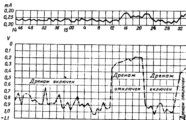
Рис. 3. Влияние дренажа кабелей АТС на плотность тока утечки водопровода.
