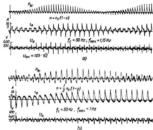
Рис. 4. Мощность, ток и напряжение на открытой фазе статора в первой a и во второй b устойчивых зонах.
