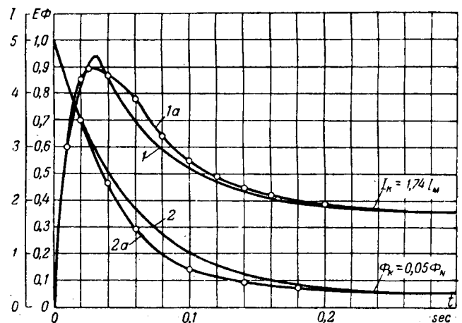
Рис. 2. Ток и поток (э. д. с.) в относительных единицах при внезапном коротком замыкании трехобмоточного генератора P_N = 4,2 \text{ kW} , U_N = 220 \text{ V} поток — \frac{\Phi}{\Phi_N} = (1 - 0,05) e^{-17,4t} + 0,05 , ток — \frac{i}{I_N} = (4,7 - 1,74) e^{-17,4t} + 1,74 .
