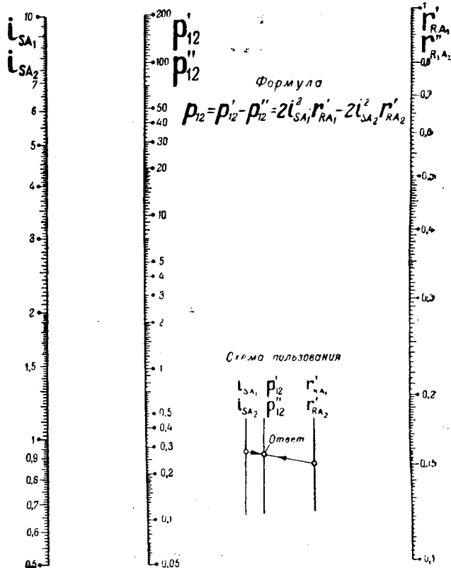
Номограмма N7
