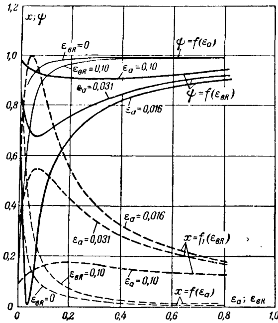
Рис. 3. Кривые x = f(\varepsilon_R) , \phi = f(\varepsilon_R) и x = f(\varepsilon_a) , \phi(\varepsilon_a) .
