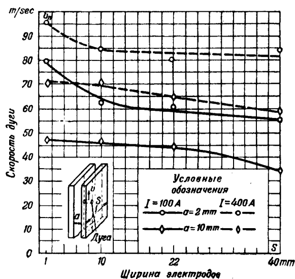
Рис. 4. Зависимость скорости движения дуги от ширины электродов при H = 800 \text{ Oe} .
