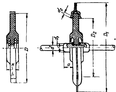
Рис. 2. Проходной изолятор дискового типа. Размеры — см. табл. 3.
