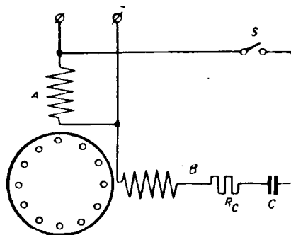
Рис. 1. Общая схема двигателя с расщепленной фазой. А — рабочая обмотка статора; В — пусковая; С — конденсатор; S — центробежный выключатель, отключающий пусковую цепь от сети при скорости 75–85% от номинальной.
