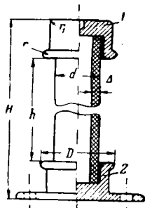
Рис. 1. Опорный изолятор.
