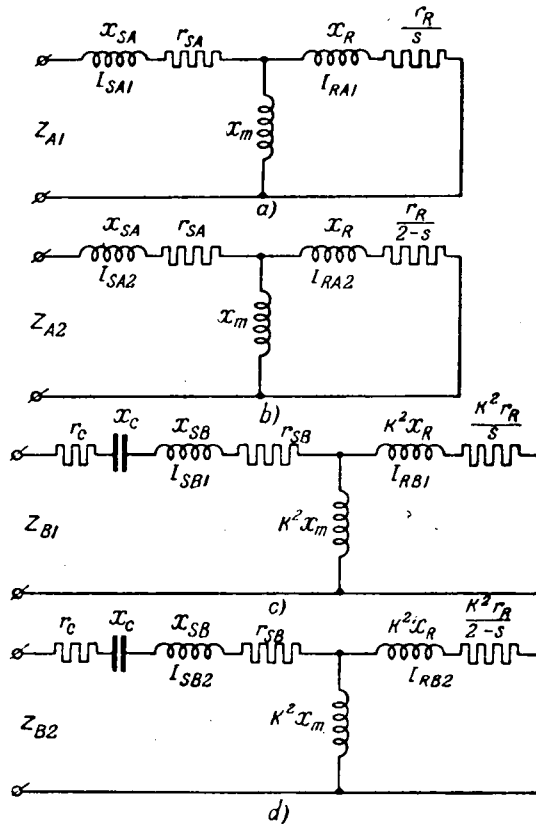
Рис. 2. Эквивалентные схемы для токов. а, в — токи прямой и обратной последовательности фазы А; с и д — то же фазы В.
