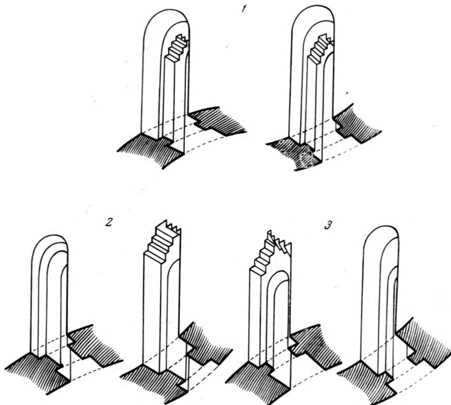
Схемы завершений оконных проемов барабанов.
