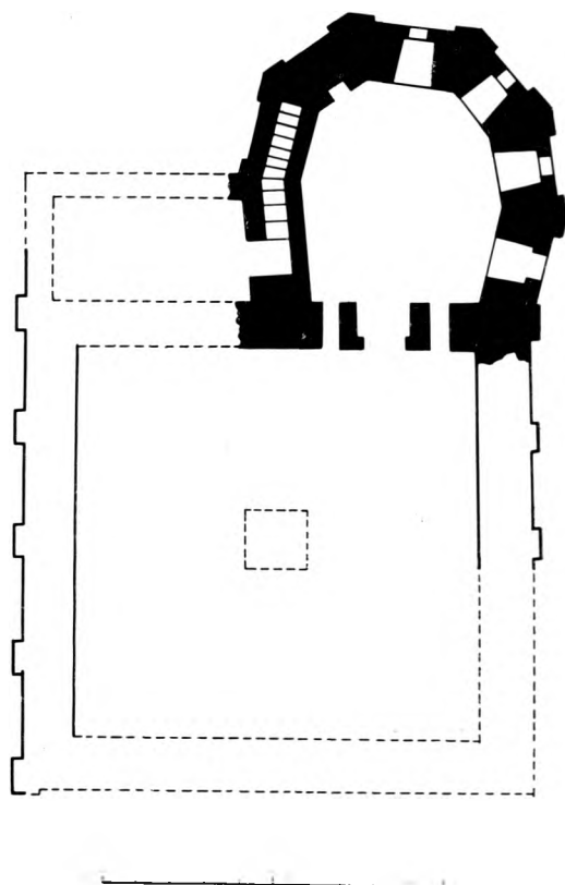
Успенская церковь и трапезная палата. Схема реконструкции плана
