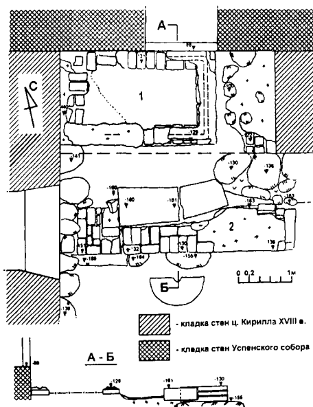
Рис. 2. Церковь Кирилла XVIII в. План расчистки в северо-западном углу храма. 1 – основание раки преподобного Кирилла; 2 – кирпичный фундамент сени над ракой.
