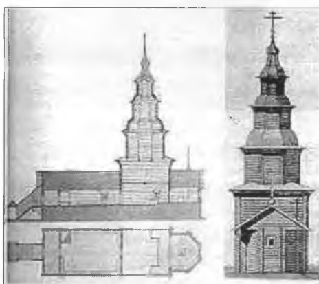
Афанасьевская Верх-Кокшеньгская церковь. Разрез, план и восточный фасад. Д. В. Милеев. Начало XX века.
