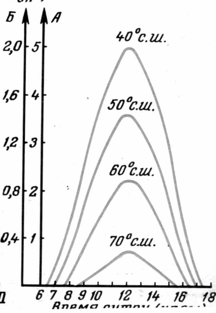
Рис. 3. Значения E_{вн}^{пас} на разных широтах 15 октября по часам.
