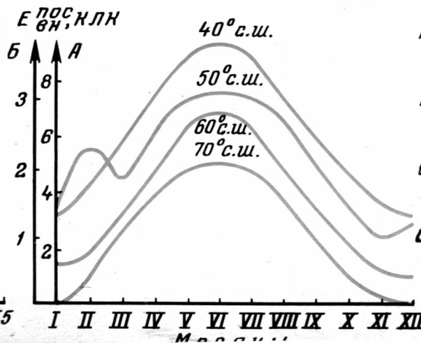
Рис. 2. Внутренняя освещенность в пасмурную погоду E_{вн}^{пас} в полдень на разных широтах по месяцам.
