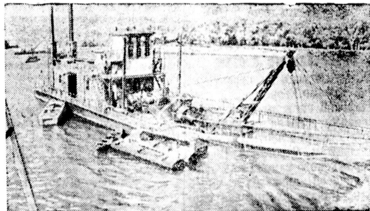
На снимке: землесосный снаряд „300-40“ № 23 в забое на рытье канала и намыве верхней перемычки котлована Каховской ГЭС. Фото Ю. Лихуты. Прессклише ТАСС.
