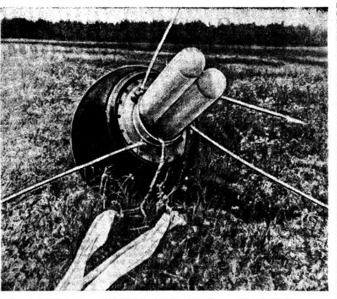
Возрастной аппарат автоматической станции «Луна-16» во время испытаний. ТАСС (Снимок принят по фототелеграфу).
