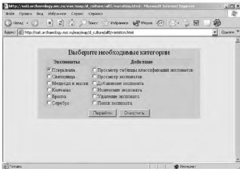
Рис. 5. Главная страница
