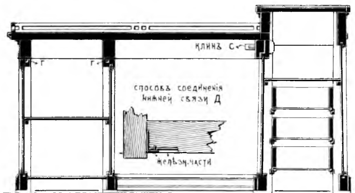
ПРОДОЛЬНЫЙ РАЗРѢЗЪ.
