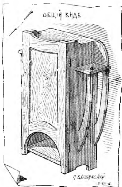
Стѣпной всячій шкафчикъ изъ сборника „Дилетантъ“.
