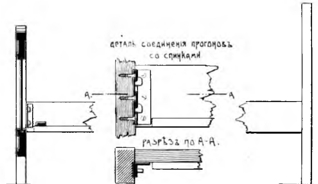
ПРОДОЛЬНЫЙ РАЗРЪЗЪ.
