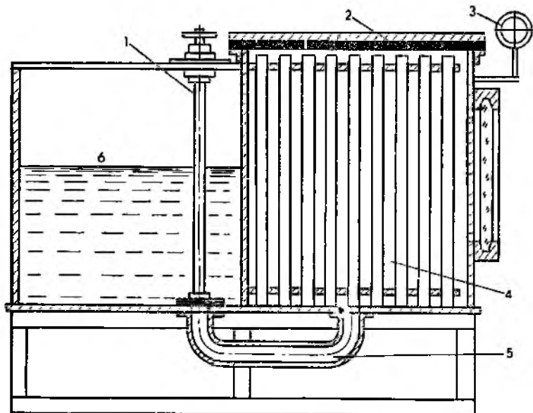
Рис. 17. Вакуумная камера для заполнения сотов искусственным кормом:
